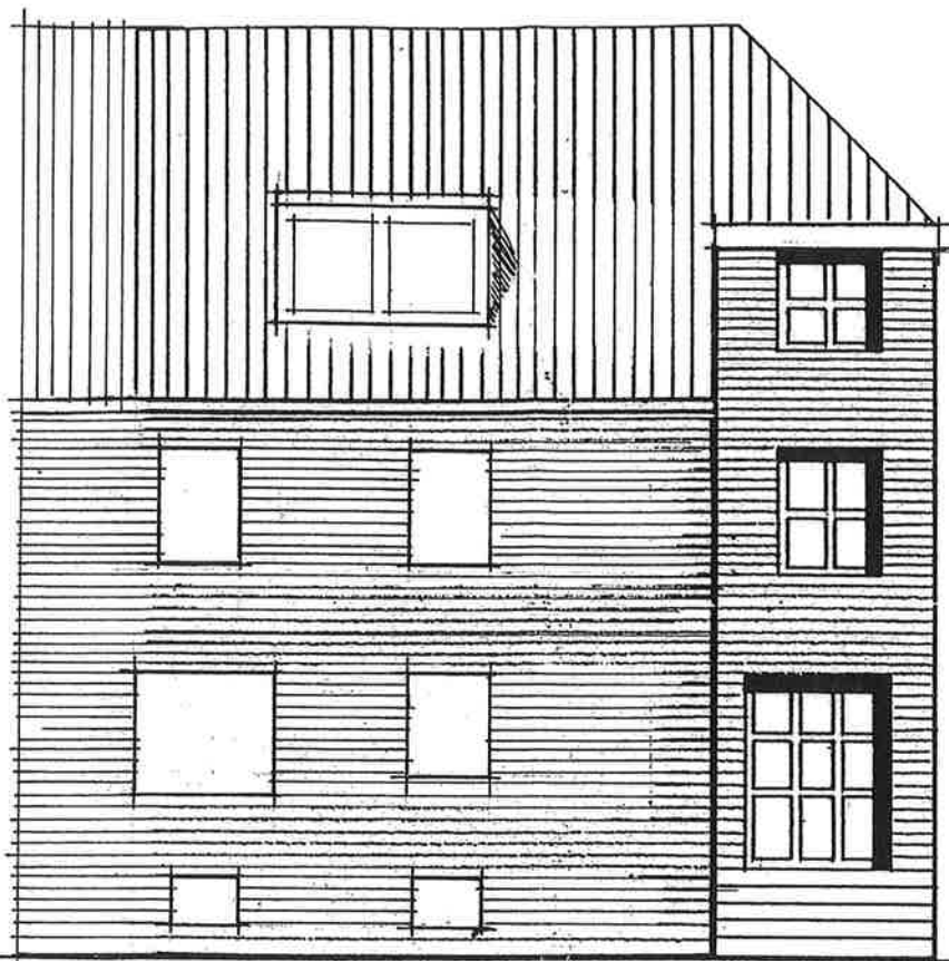
STRASSENANSICHT
