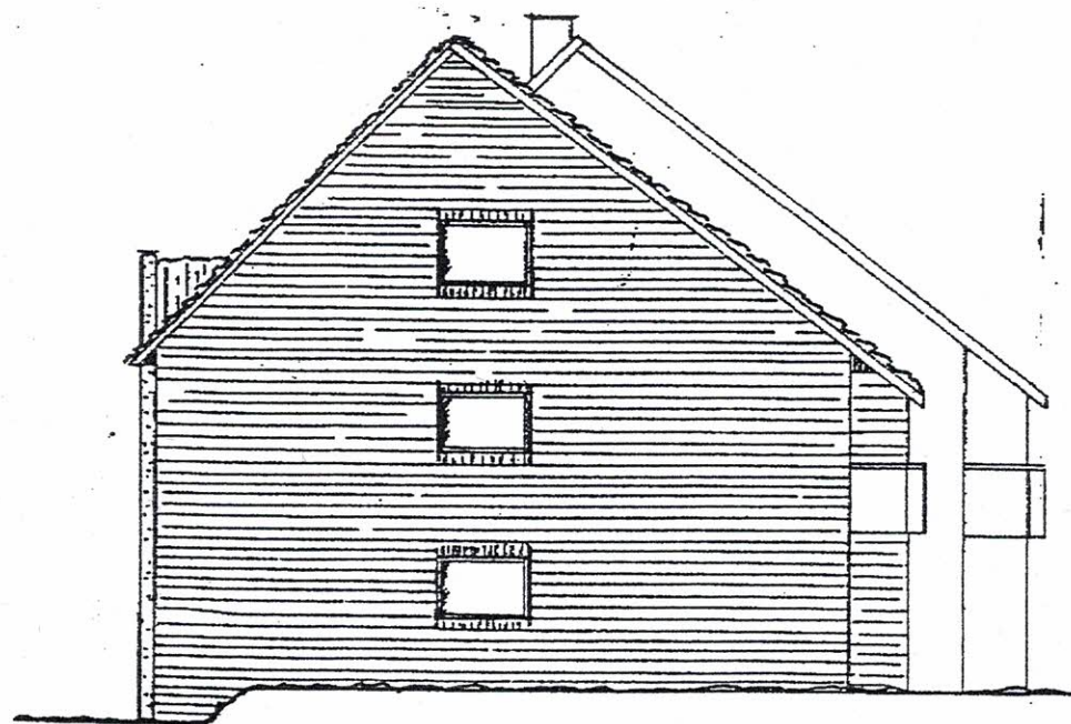
Südansicht
