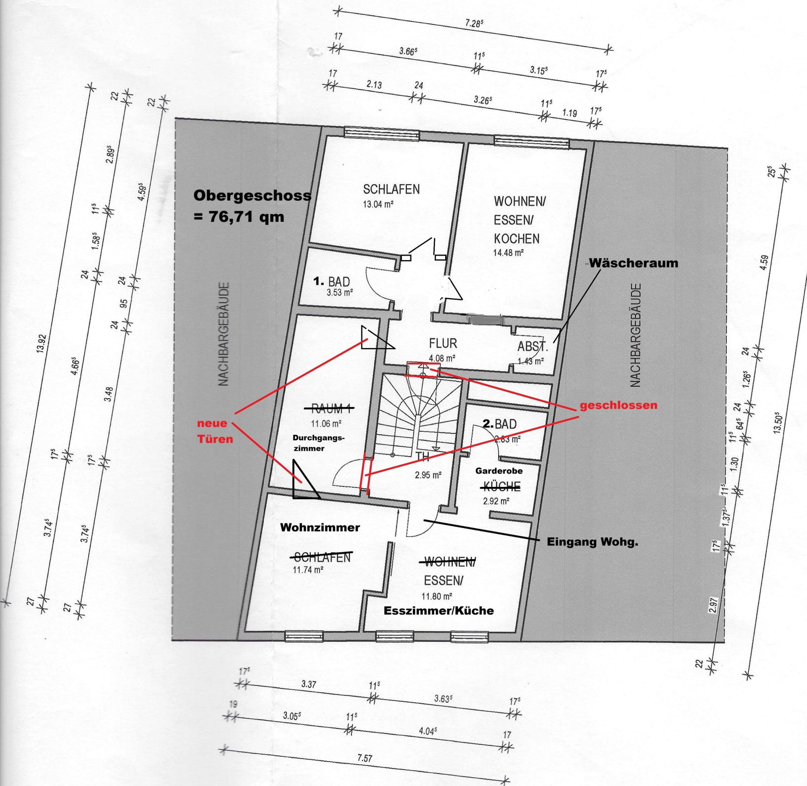
OBERGESCHOSS EBENE +2,70/+2,19
