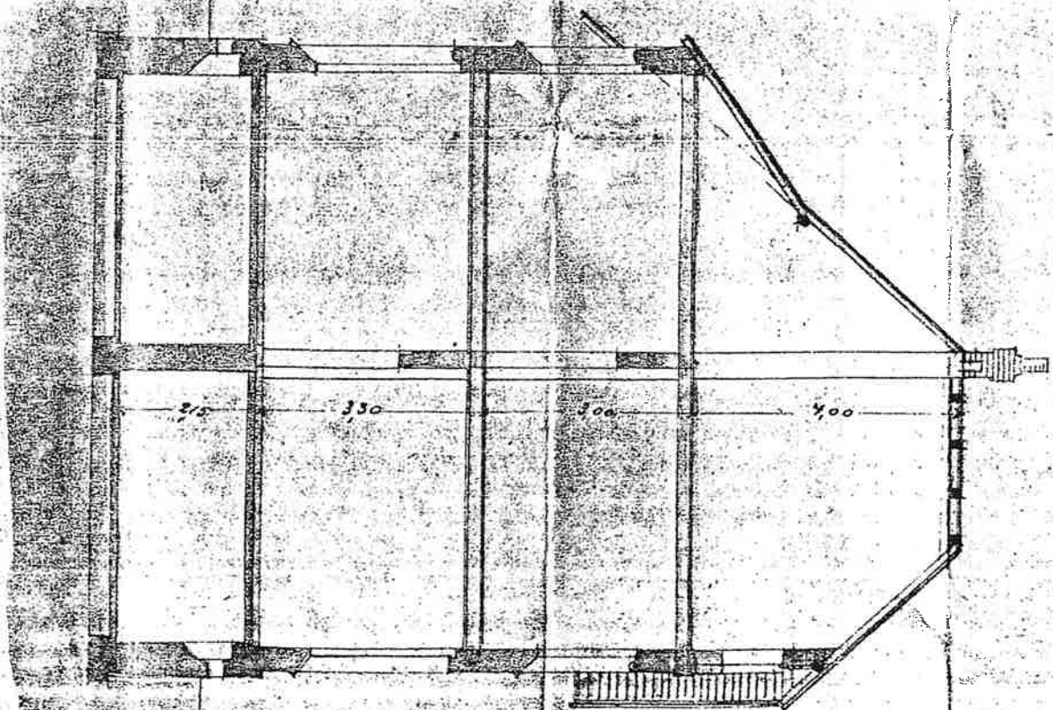
SCHNITT E-F
