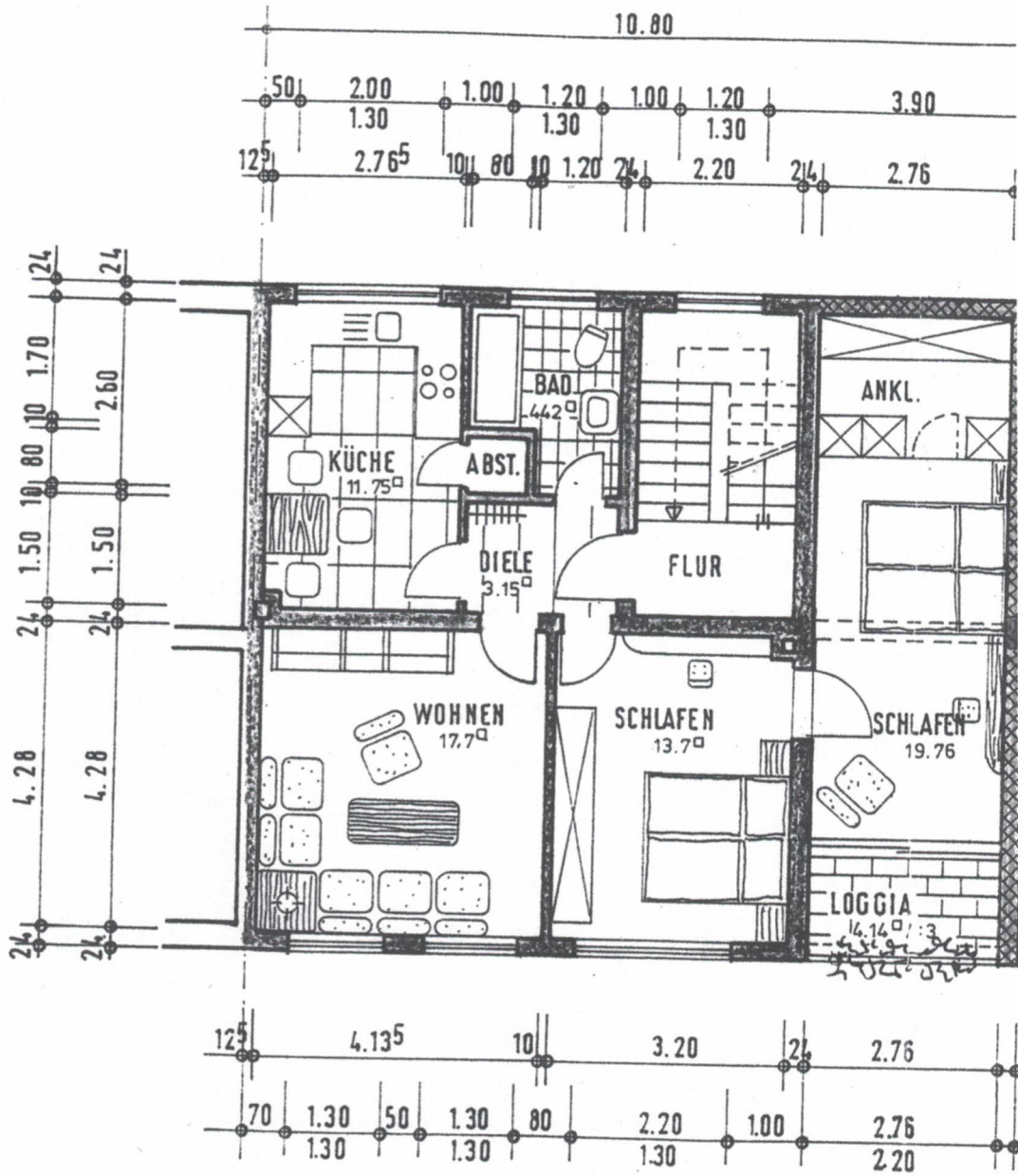
1.+ 2. OBERGESCHOSS ( NEUGEPLANT )
