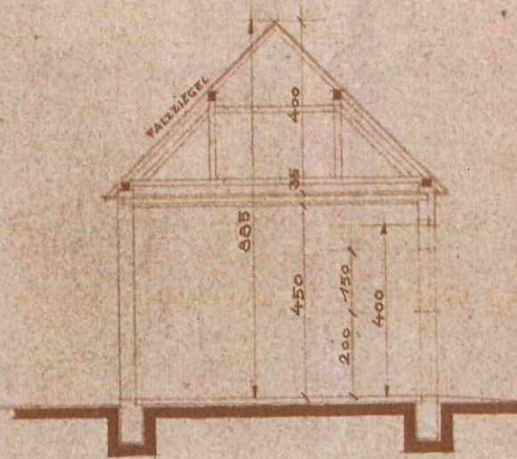
SCHNITT A-B
