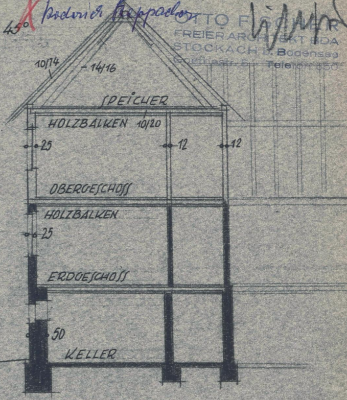
QUERSCHNITT M. 1:100
