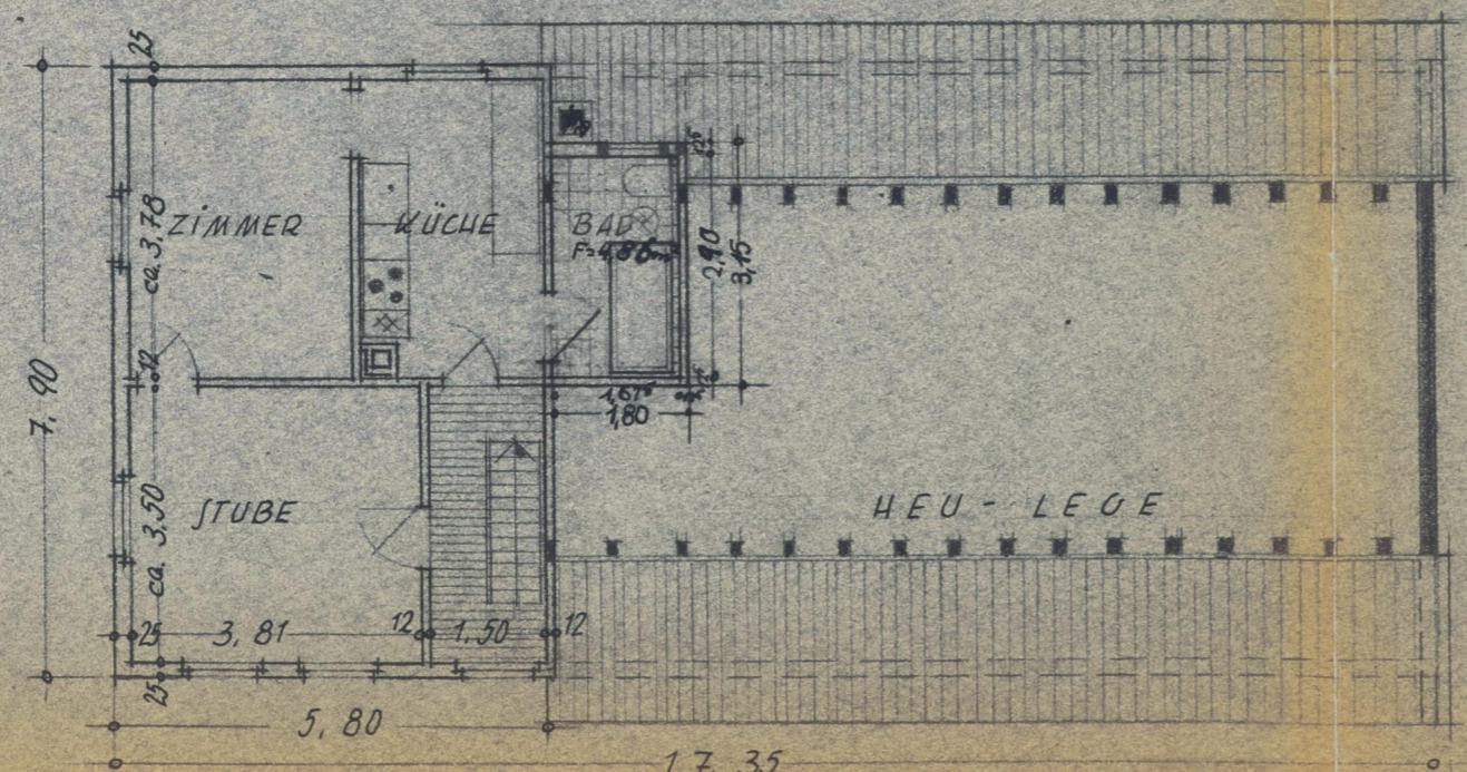
OBERGESCHOSS M. 1:100
