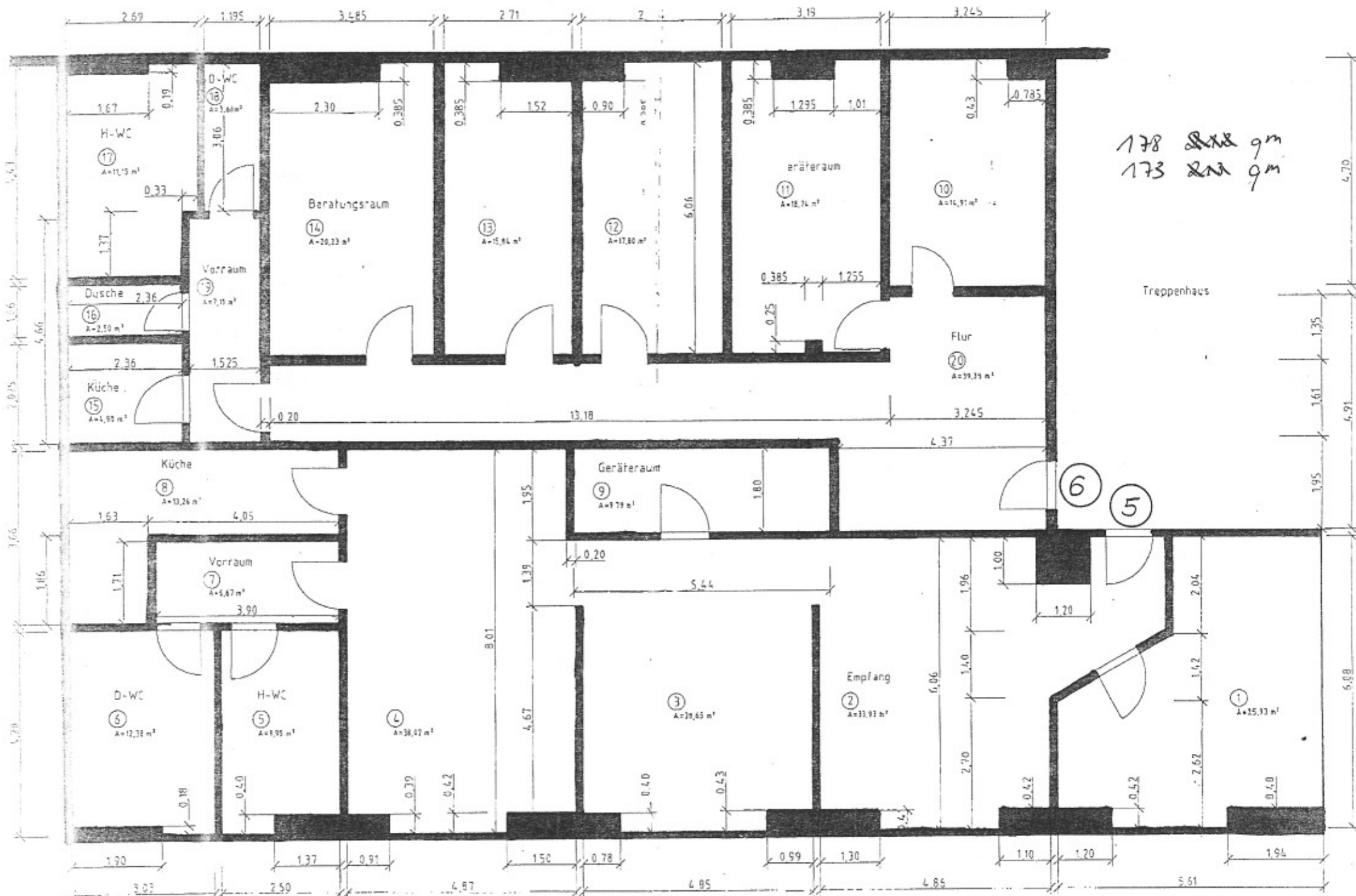
Grundriss 2.OG li/re Gewerbeeinheit
