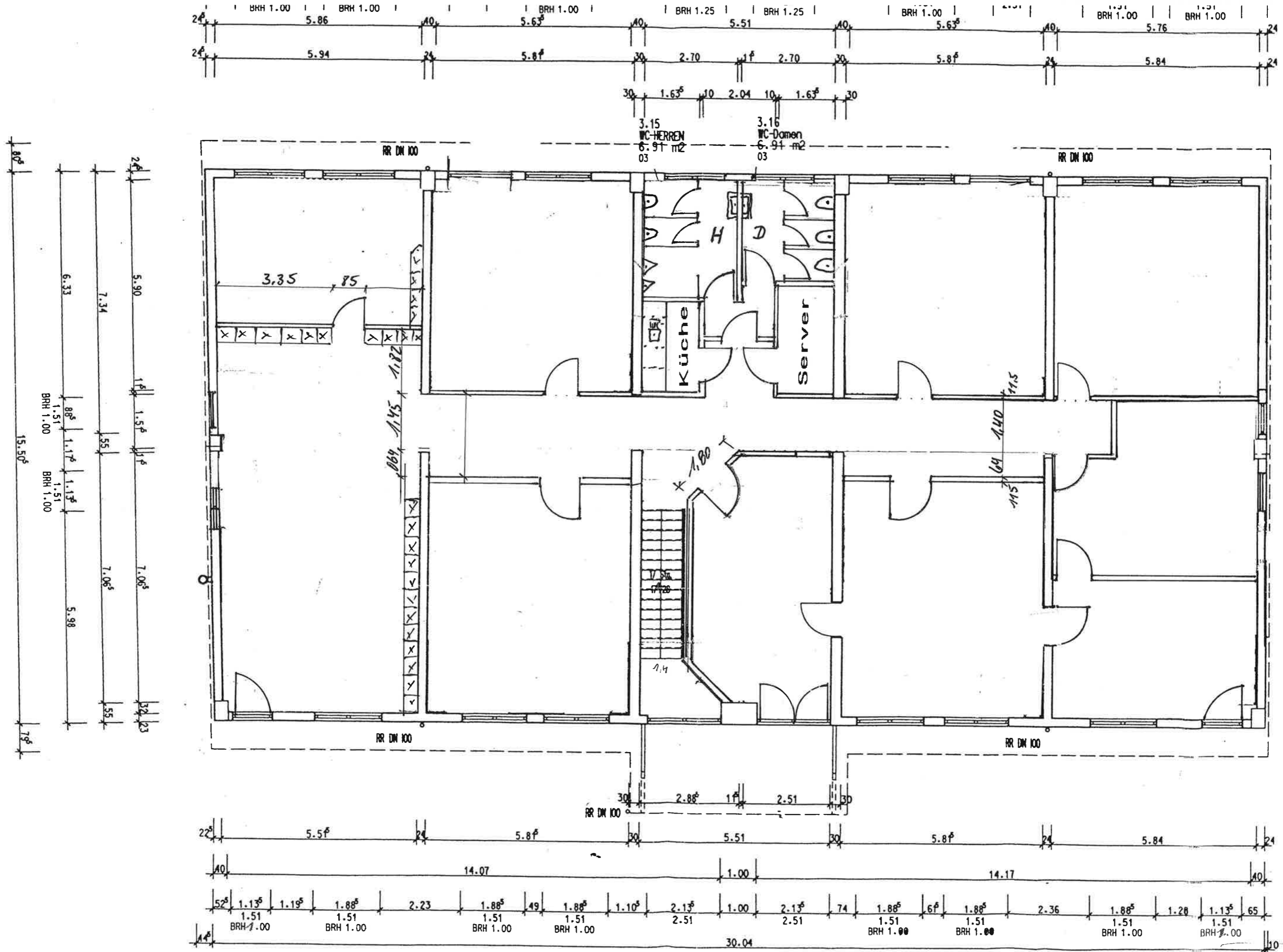
67346 Speyer Ziegelofenweg 46 d Obergeschoß M: 1/100
