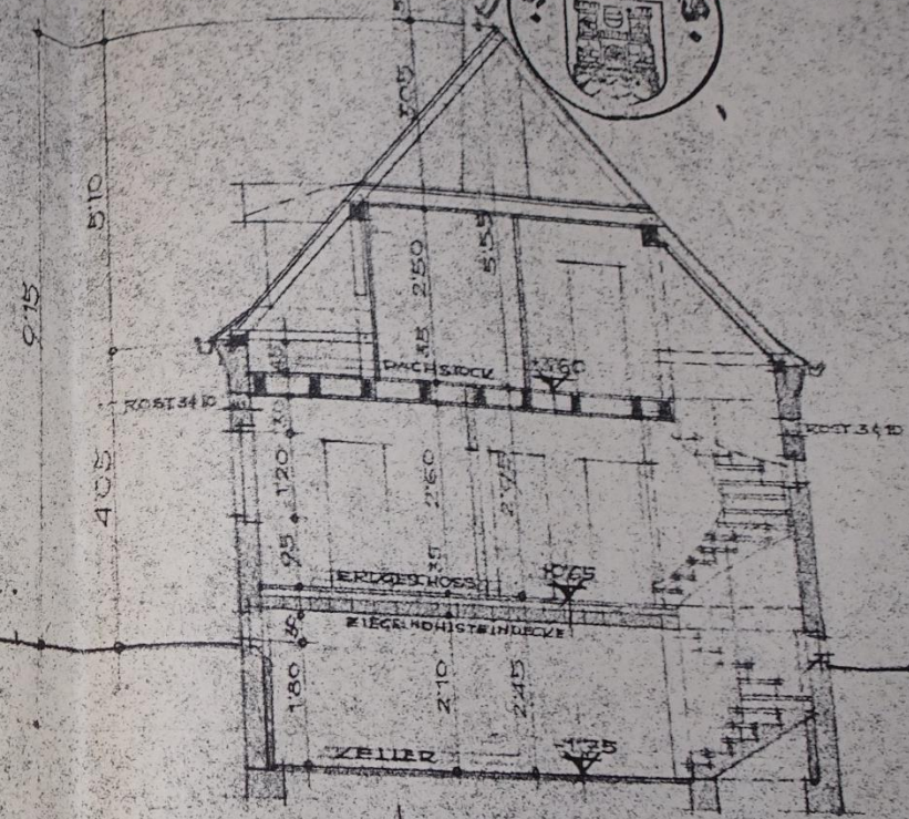
SCHNITT A-B.
