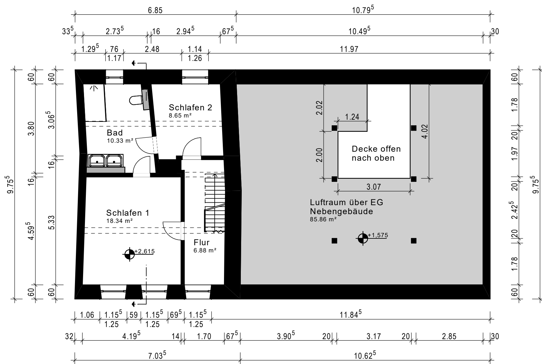
Obergeschoss
