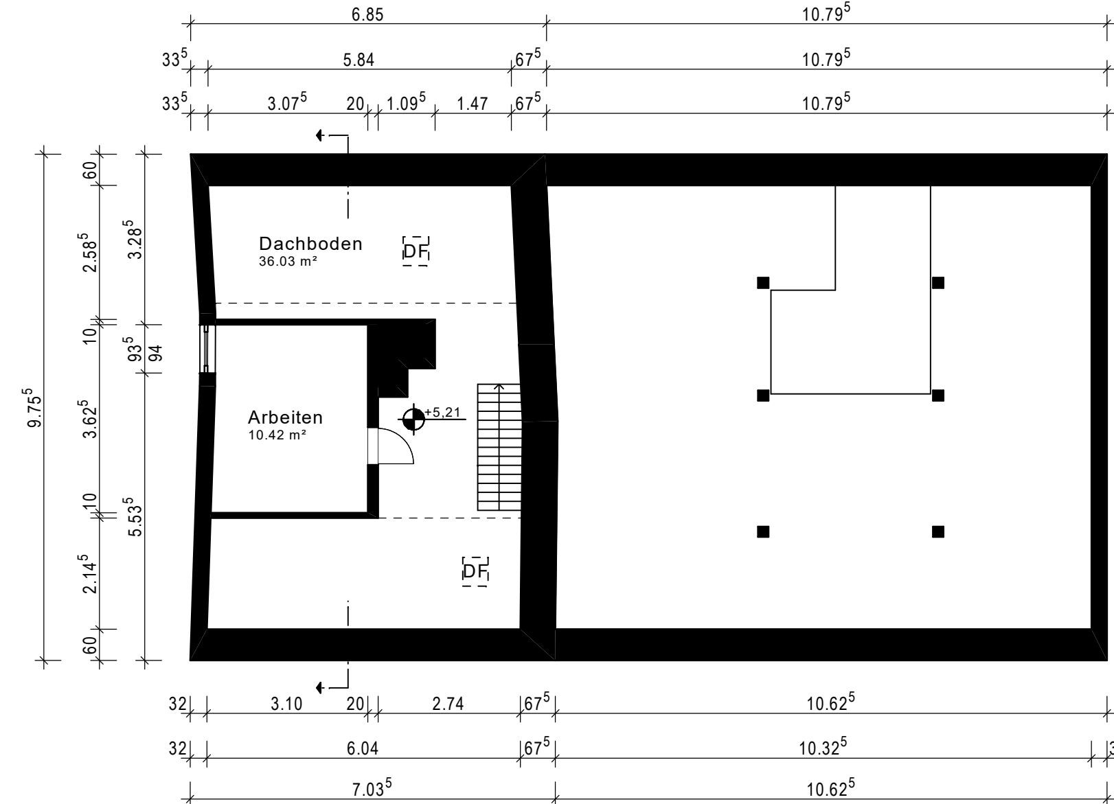
Dachgeschoss
