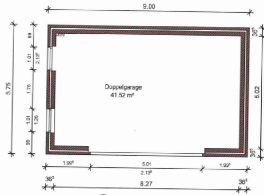
Grundriss
