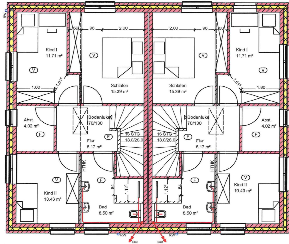
Dachgeschossgrundriss
