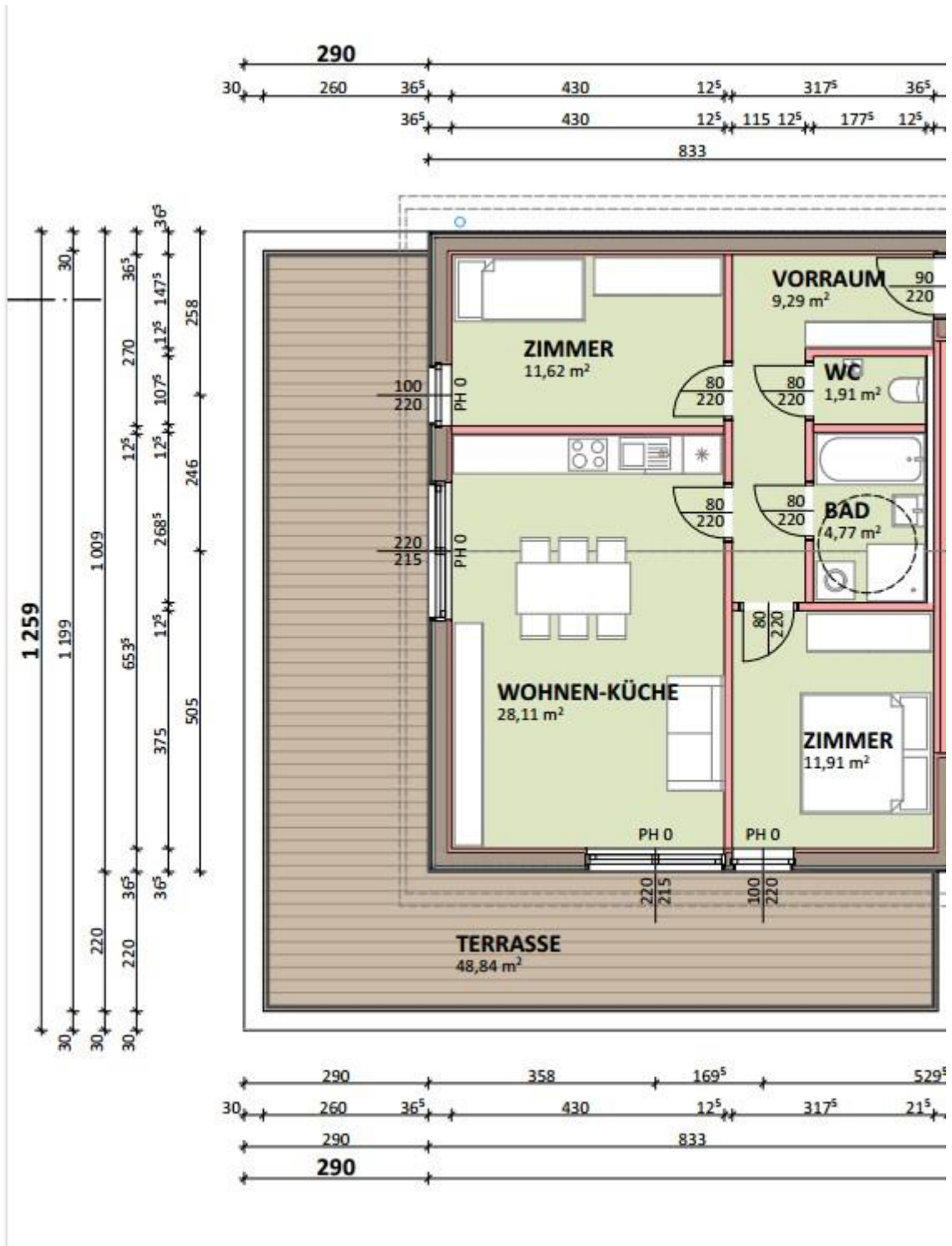
Bemaßter Grundriss TOP 1
