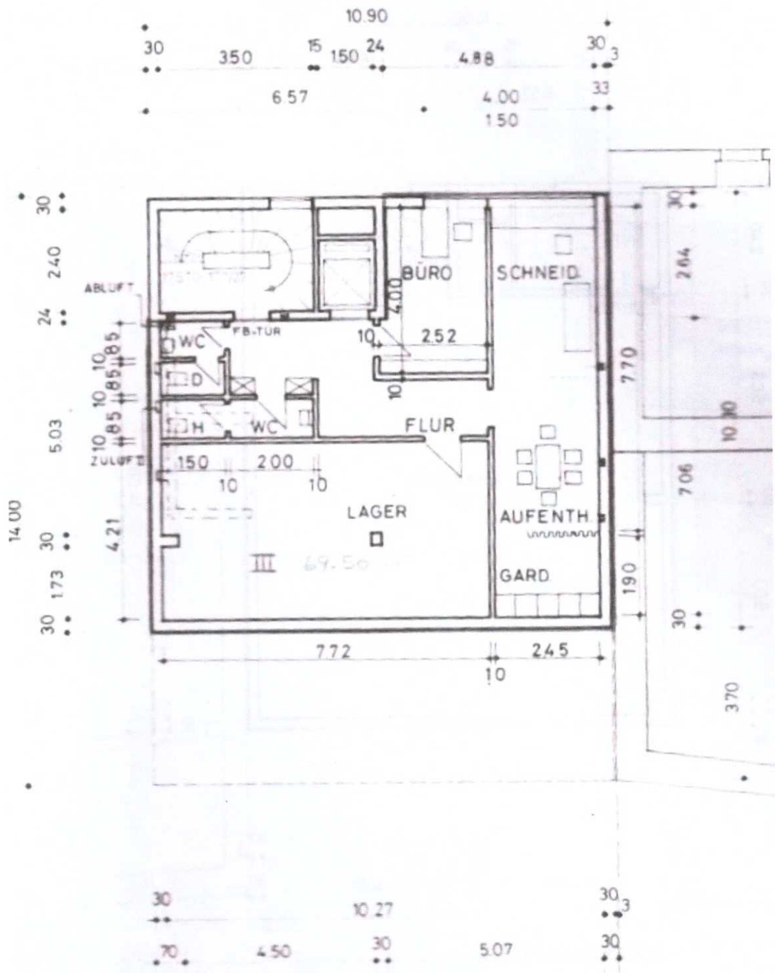
2. UNTERGESCHOSS
