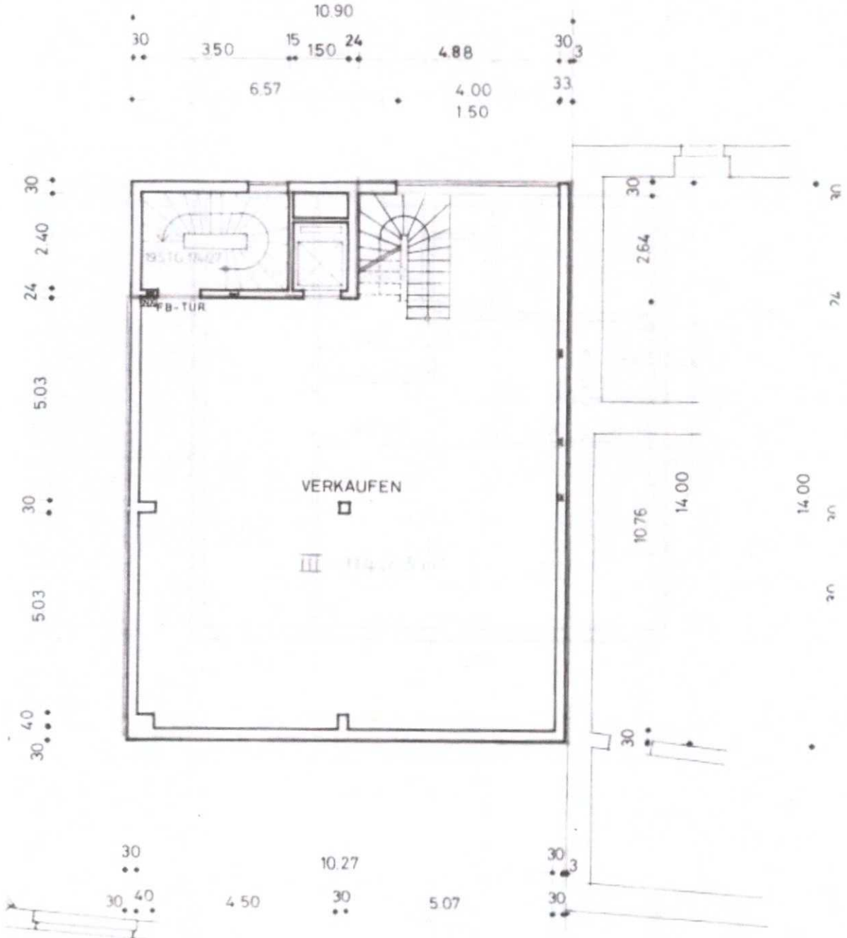
1. UNTERGESCHOSS
