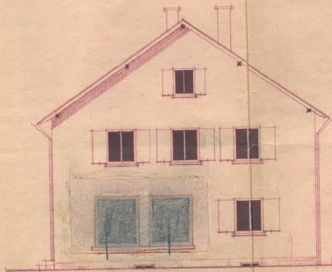
Nord-Ansicht
