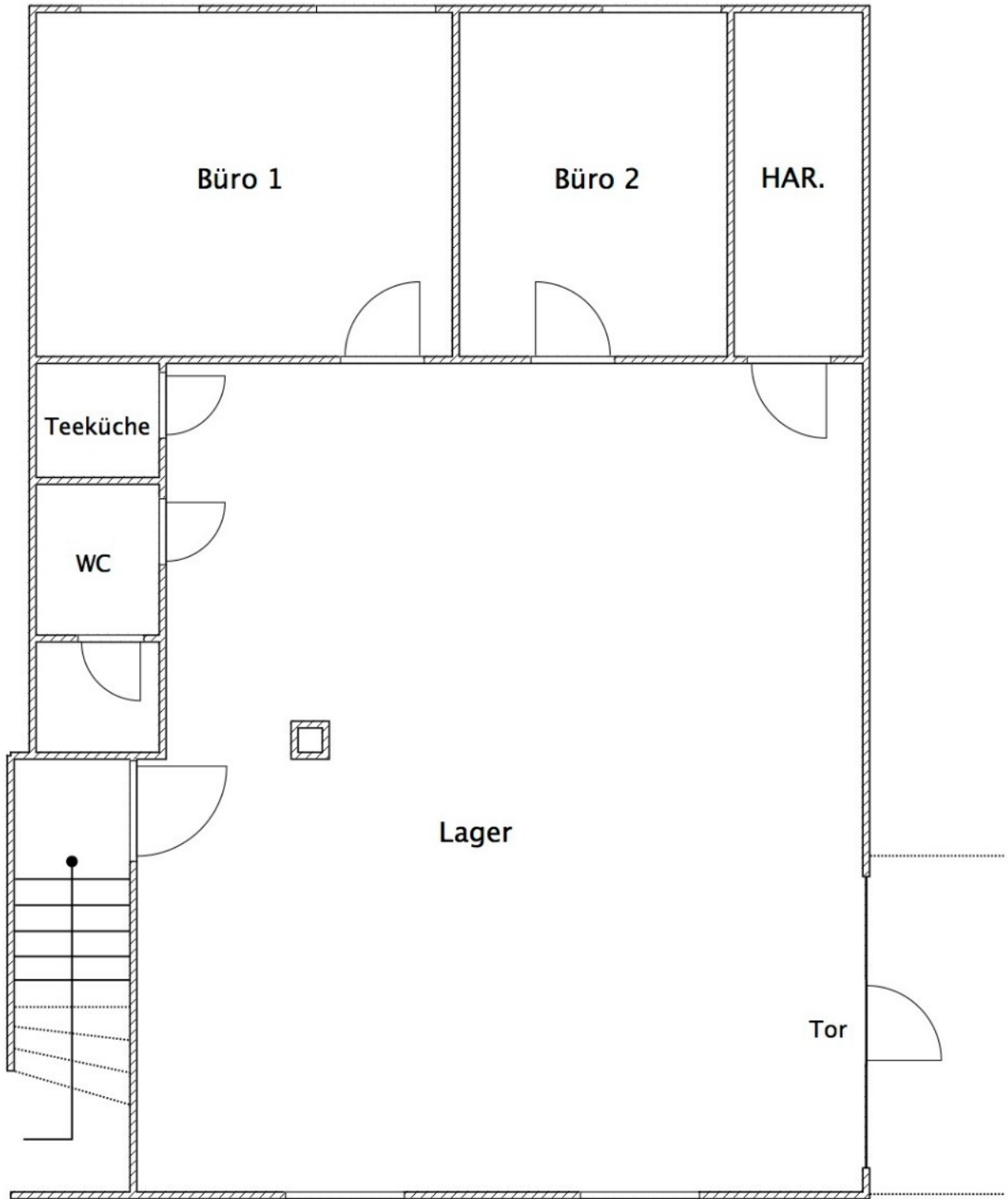
Grundriss Skizze UG
