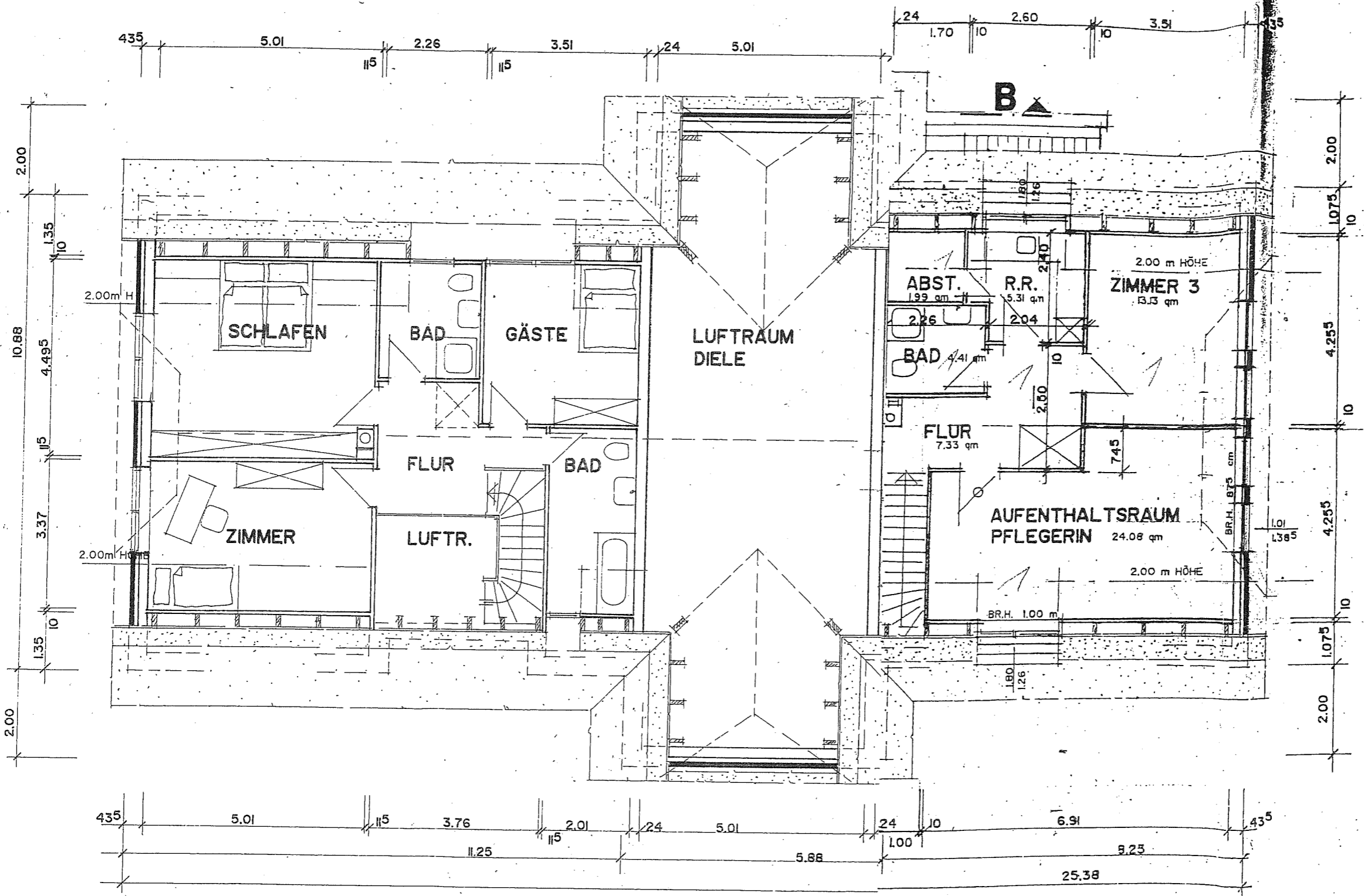
GRUNDRISS : DACHGESCHOSS , M. 1 : 100
