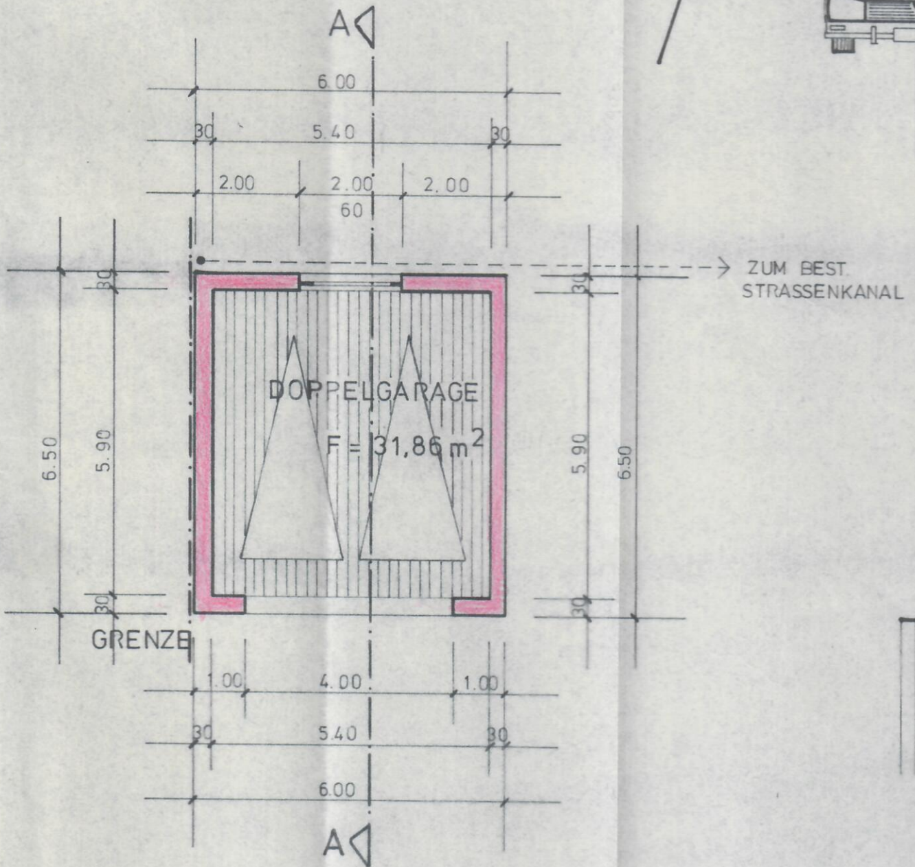
GRUNDRISS
