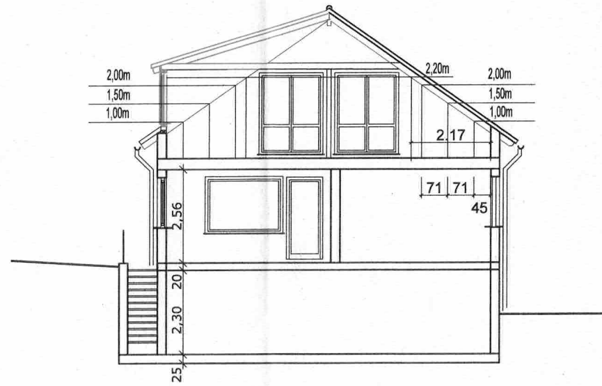
Schnitt B-B
