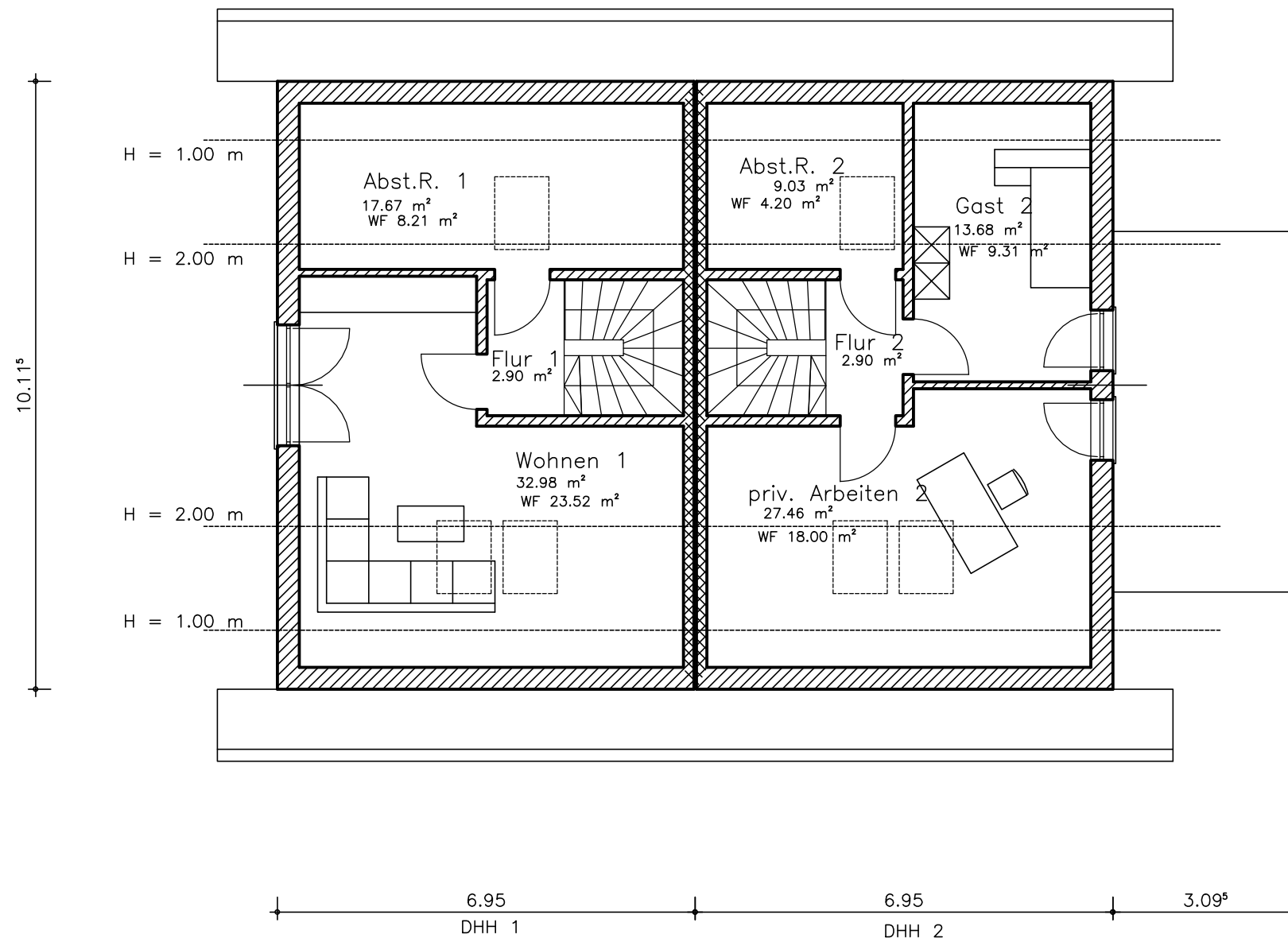
Dachgeschoss – Grundriss
