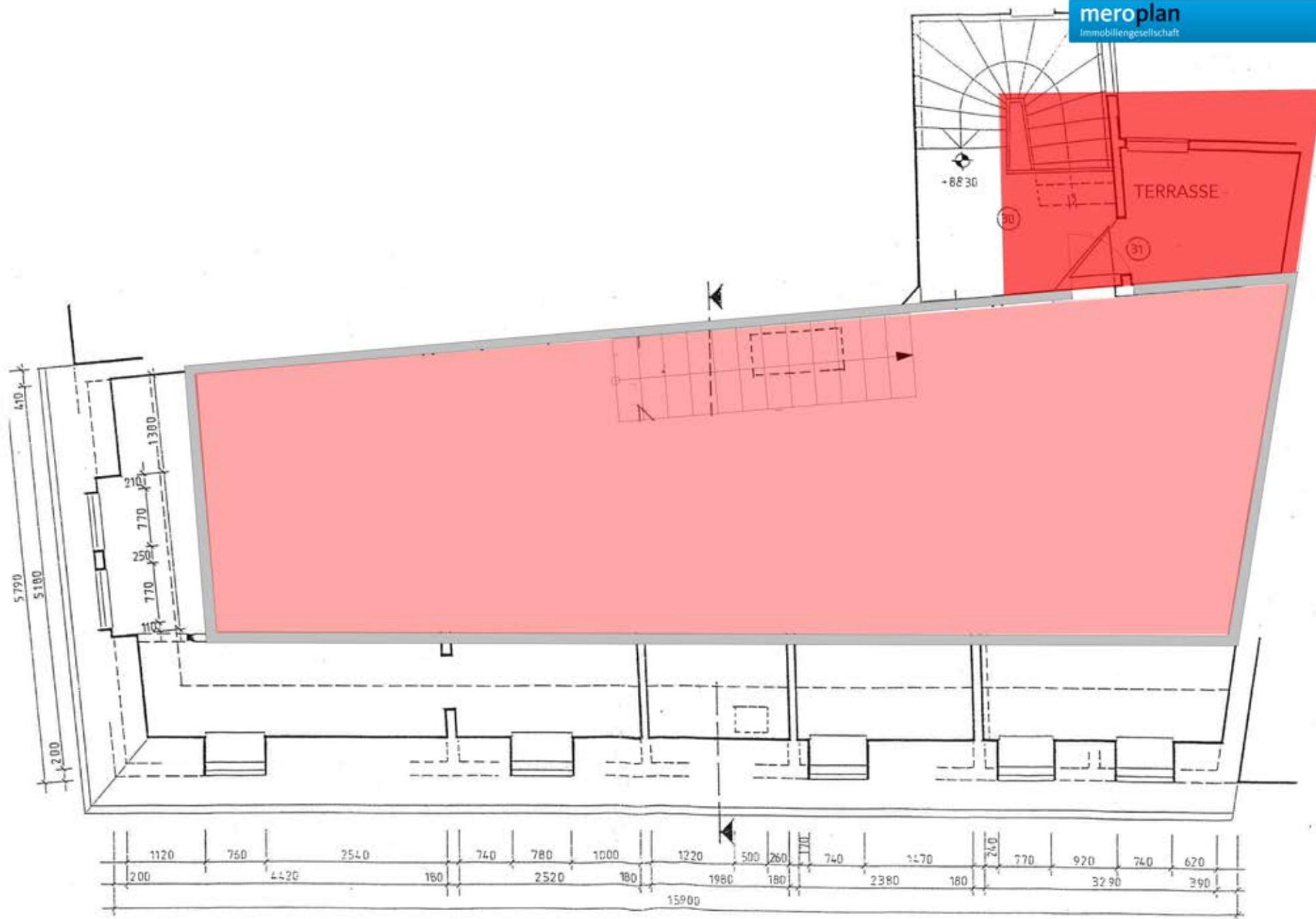
GRUNDRISS MANSARDGESCHOSS SCHNITTEBENE BRÜSTUNGSHÖHE 760 MM
