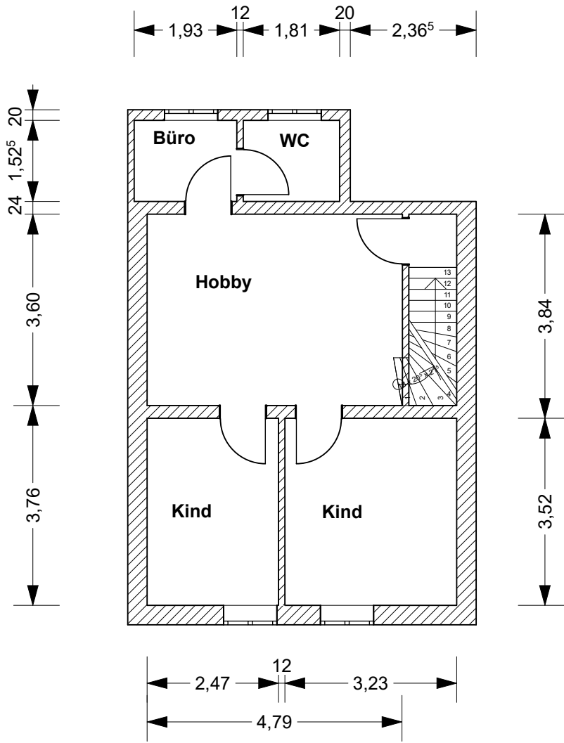
Obergeschoss
