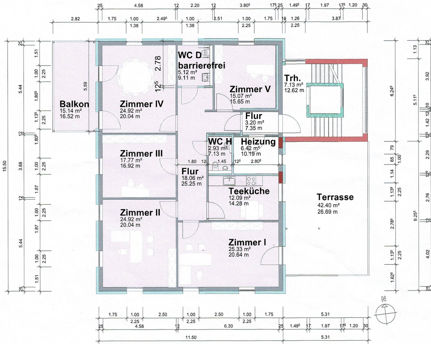
1. Obergeschoss
