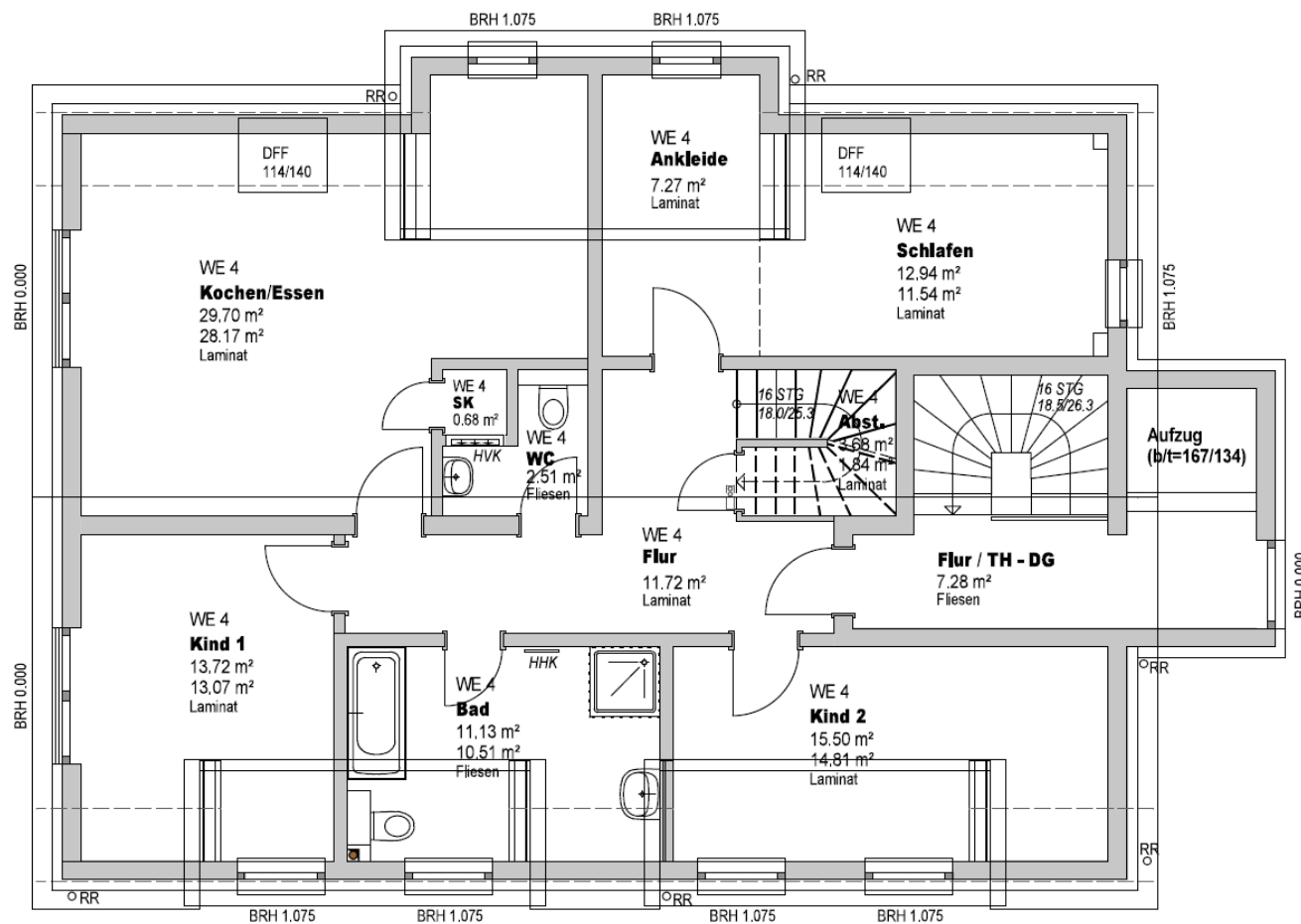
Grundriss 1. Dachgeschoss
