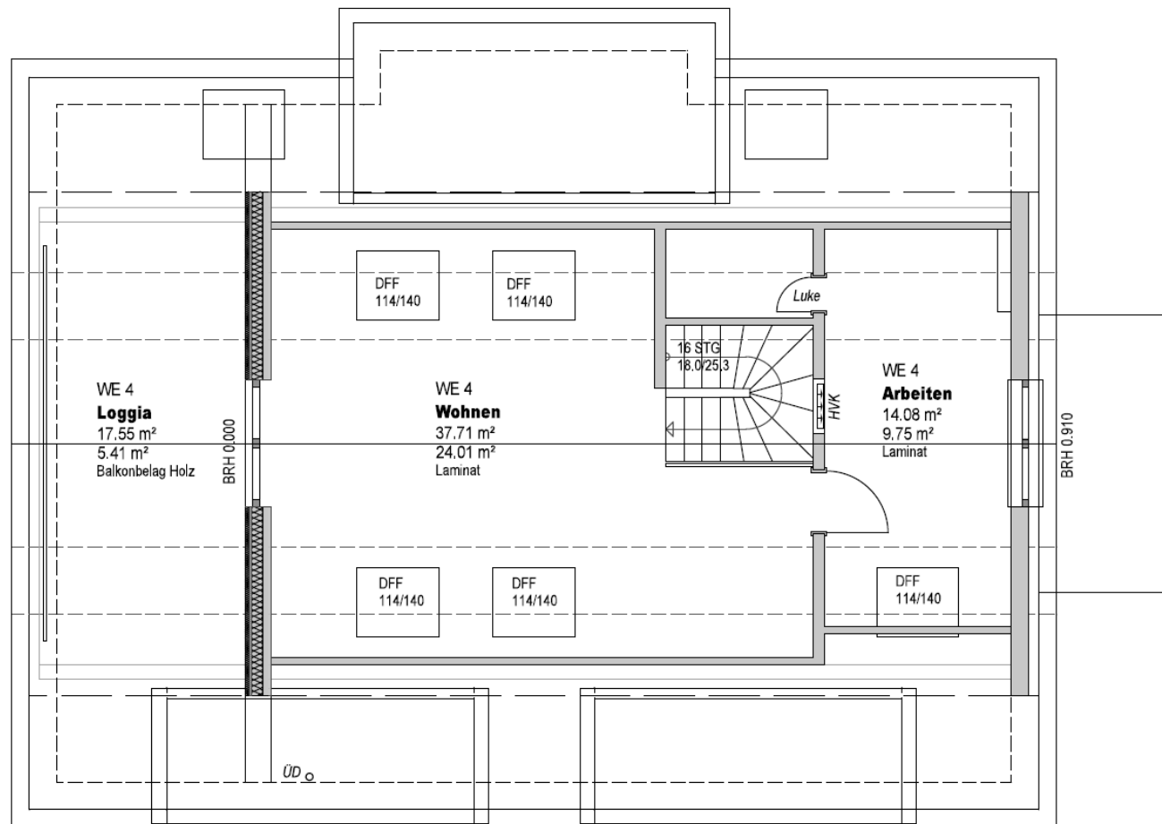
Grundriss 2. Dachgeschoss
