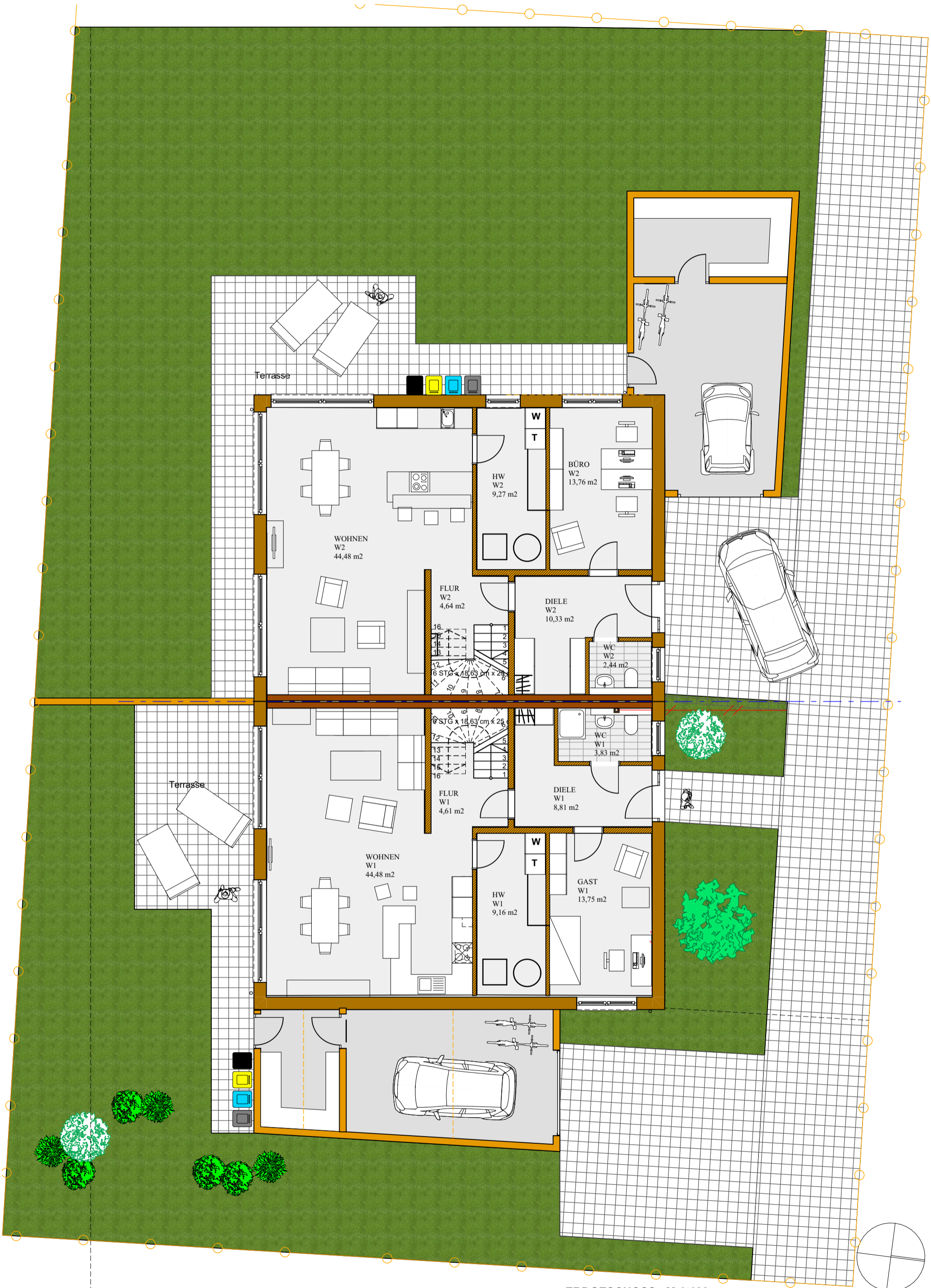
ERDGESCHOSS M 1:100
