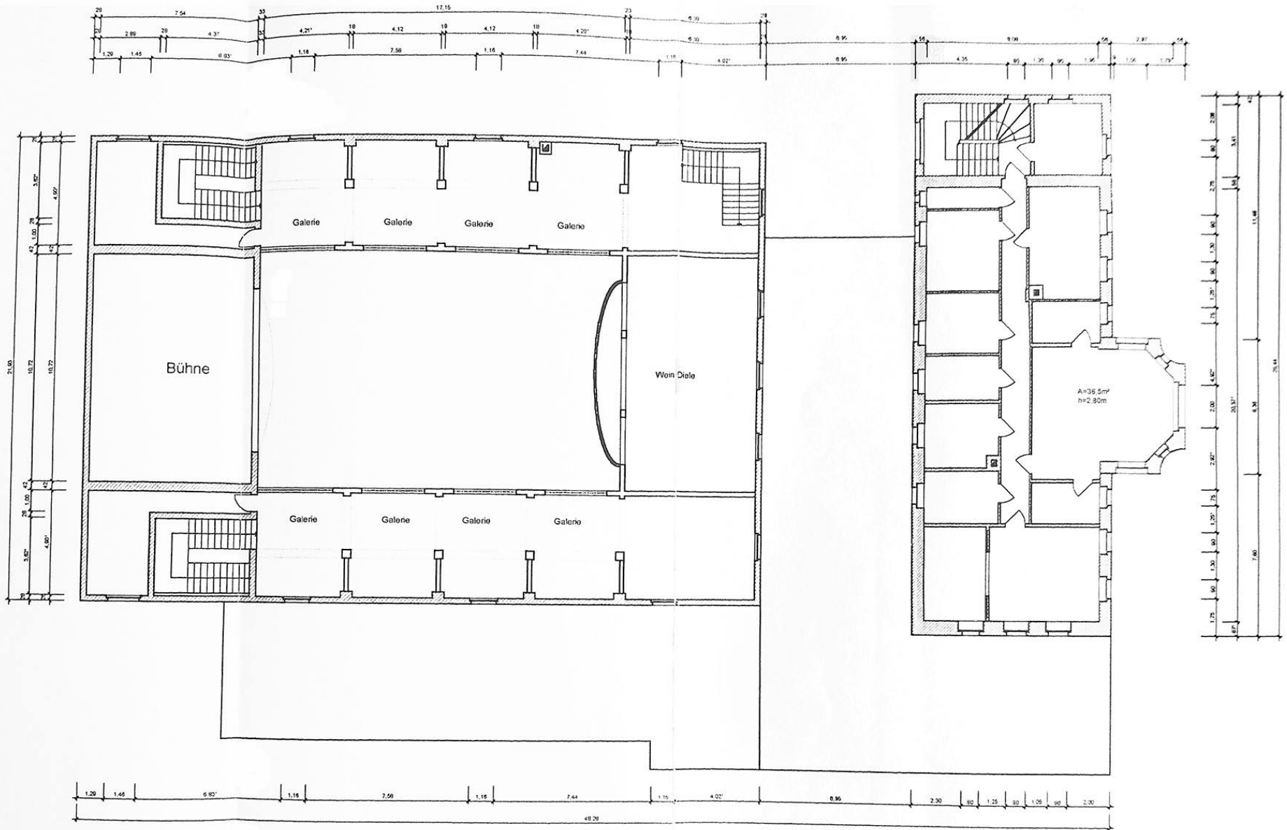
Grundriss 1. Obergeschoss
