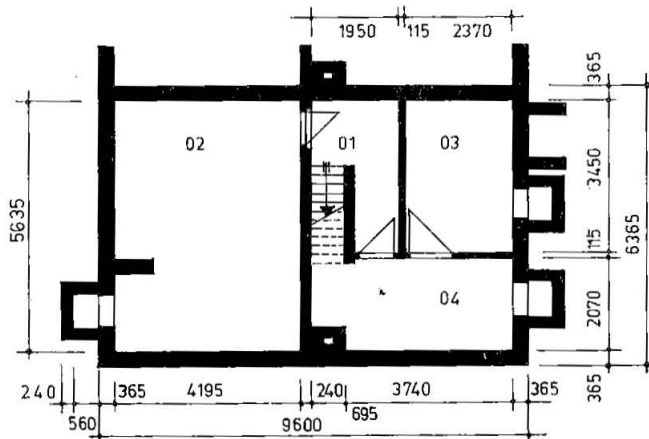
KELLERGESCHOSS
