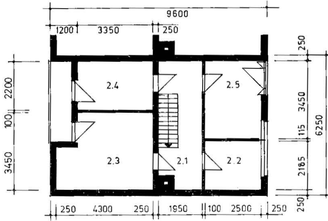
OBERGESCHOSS
