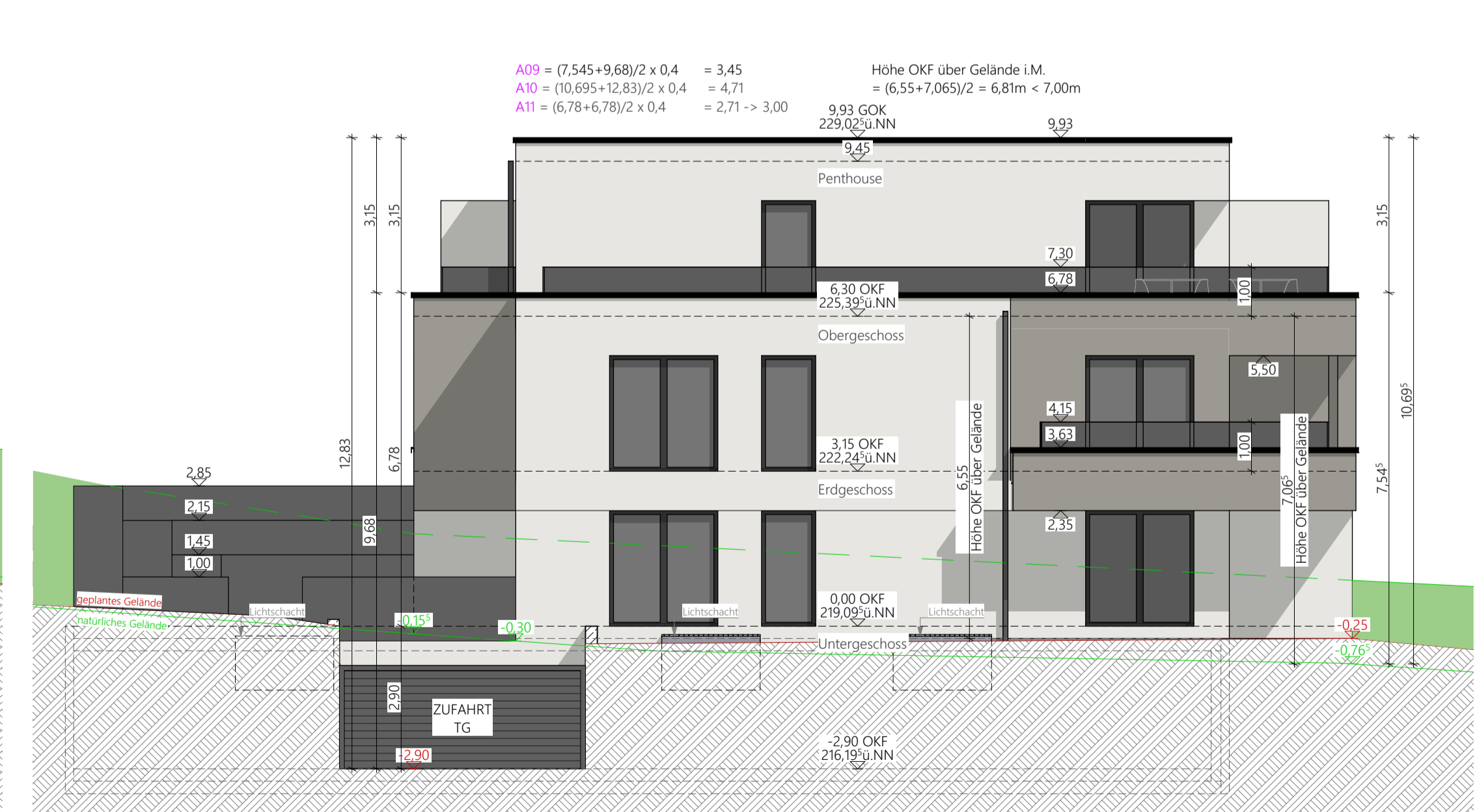
ANSICHT NORD
