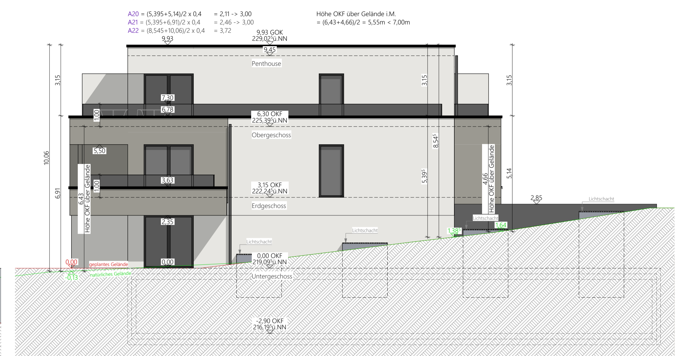
ANSICHT SÜD
