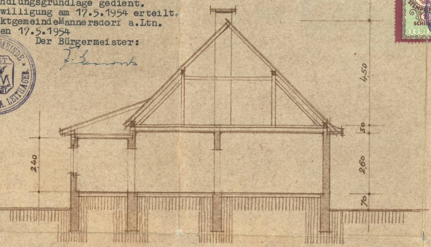
SCHNITT A-B
