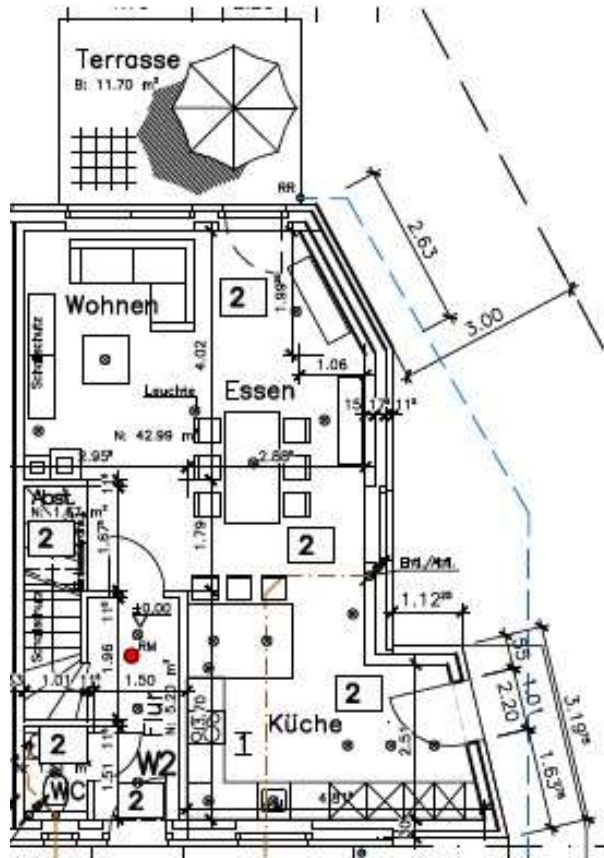
Grundriss Erdgeschoss
