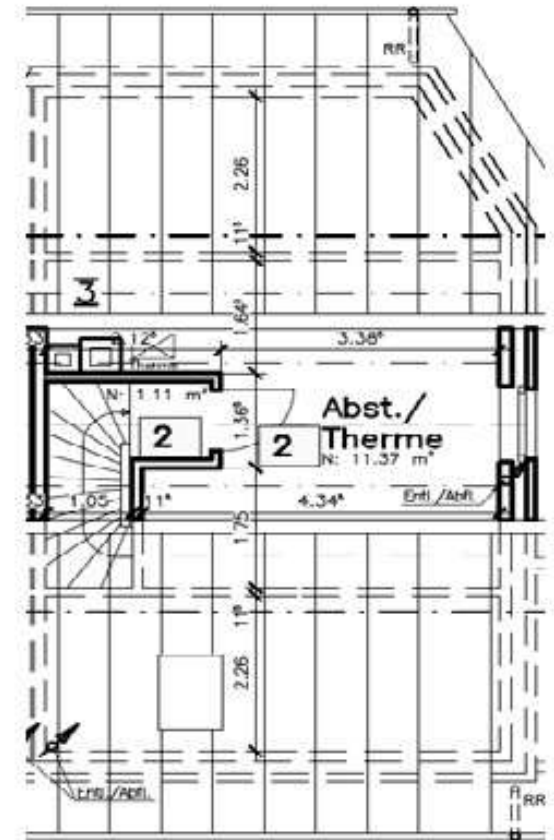
Grundriss Dachgeschoss
