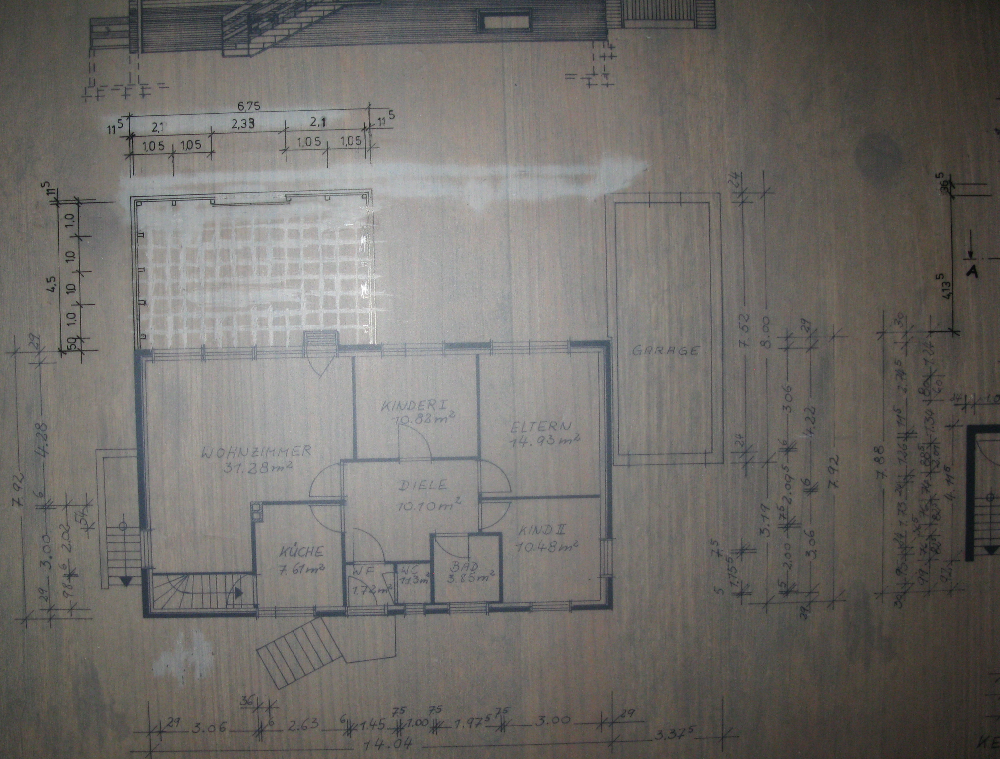
ERDGESCHOSS
