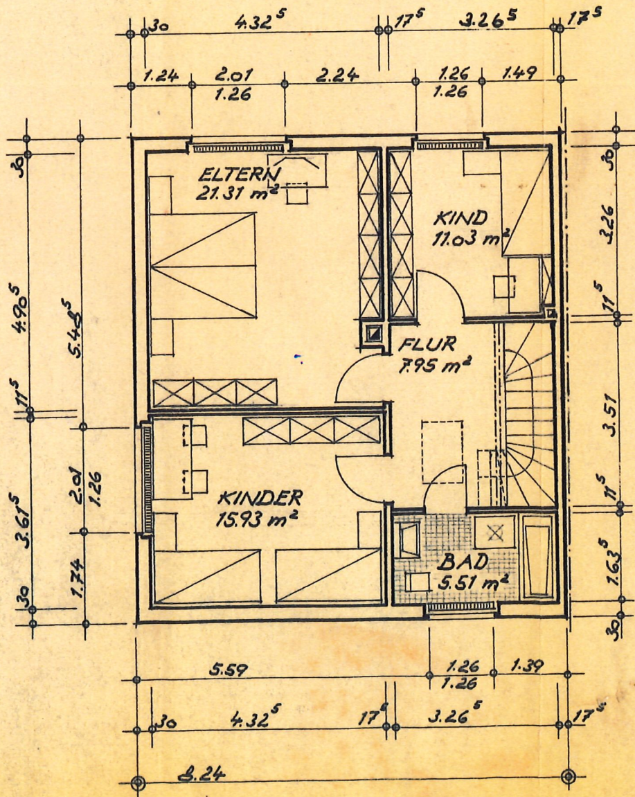
OBERGESCHOSS
