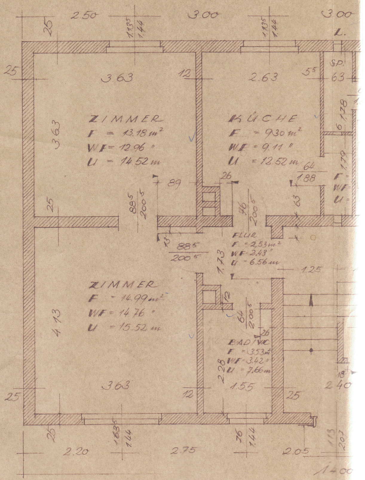
ERD- U. 1. OBERGESCHOSS
