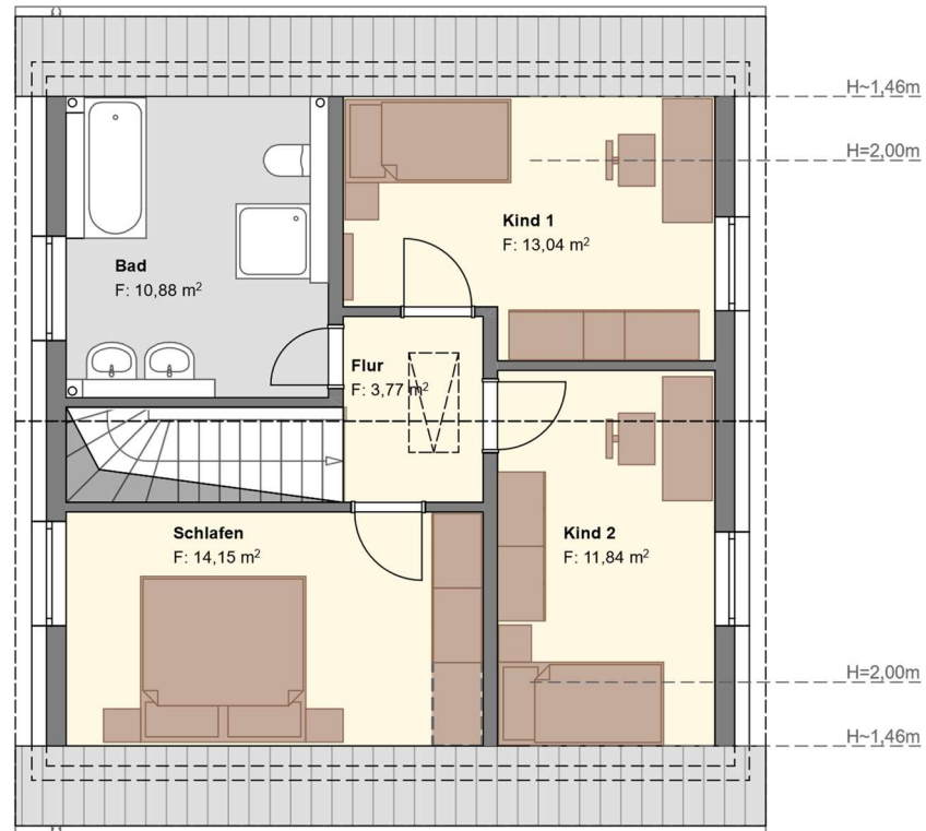
Obergeschoss family 112 grün
