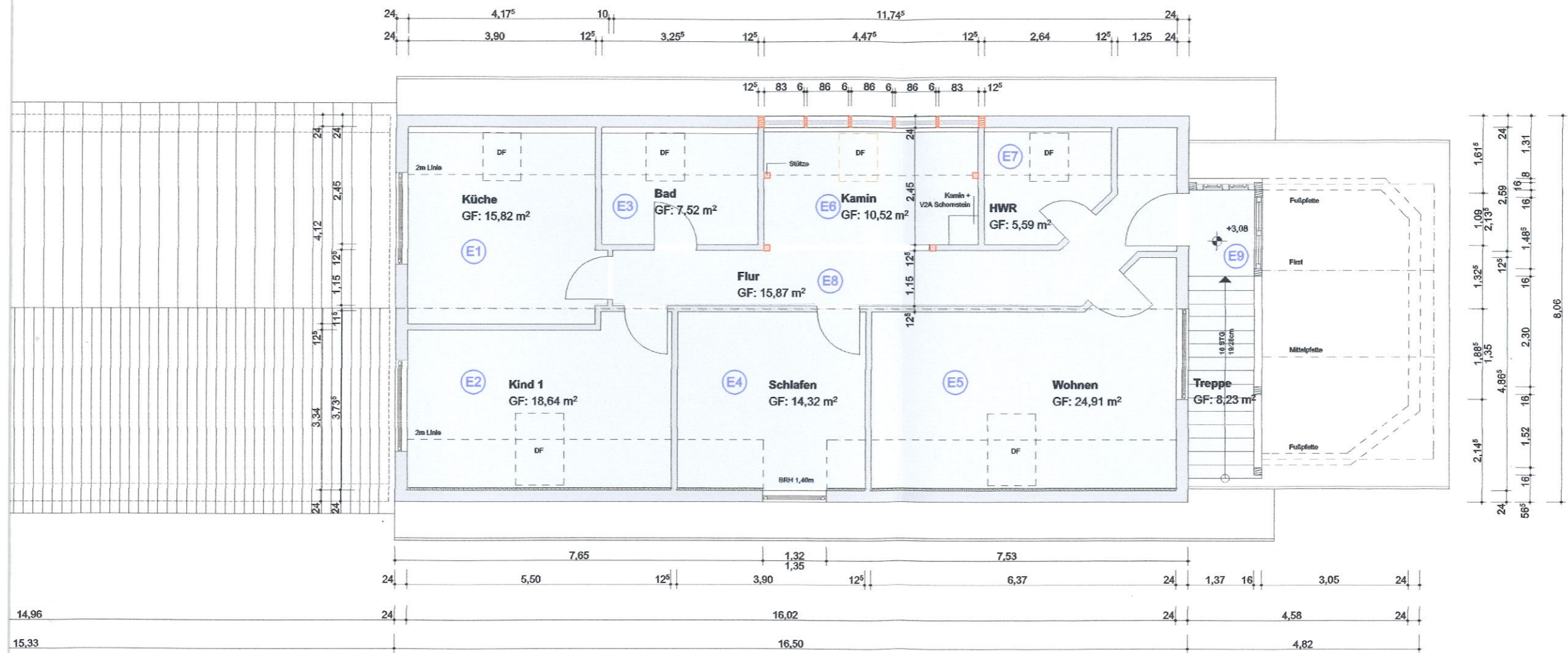
GRUNDRISS OBERGESCHOSS
