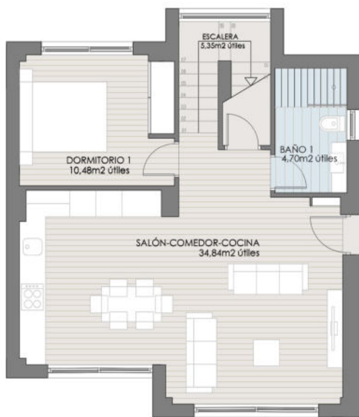
PLANTA BAJA E: 1/75
