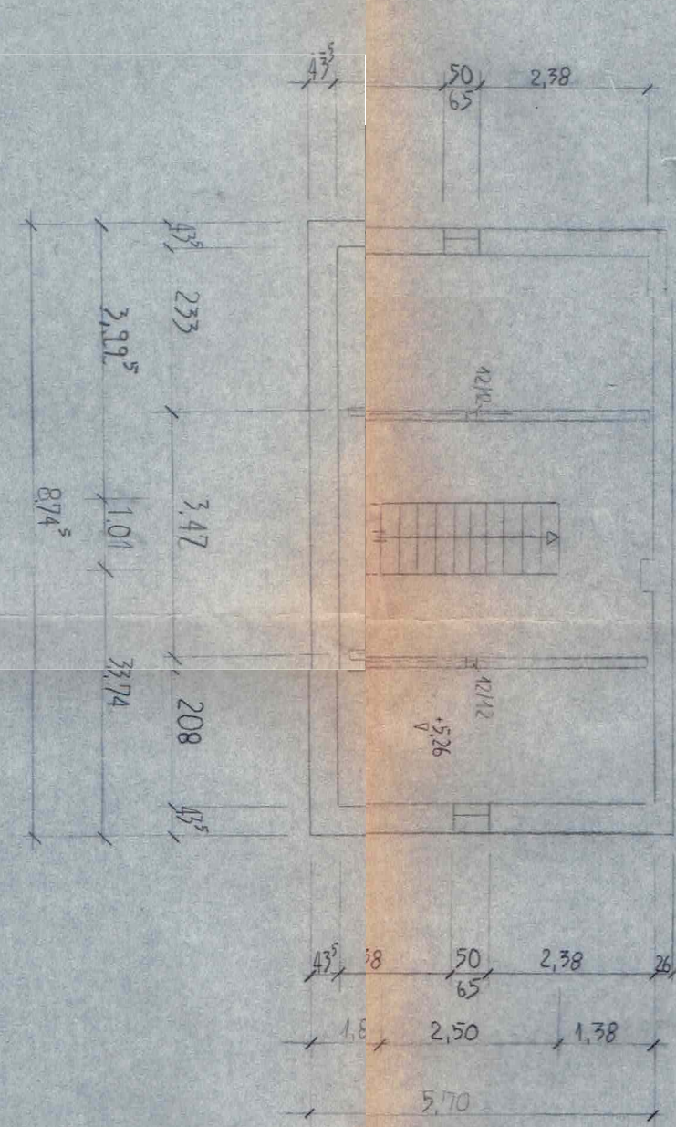
OBERGESCHOSS
