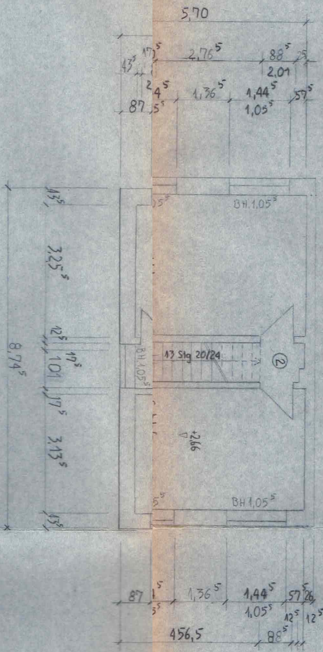
ERDGESCHOSS
