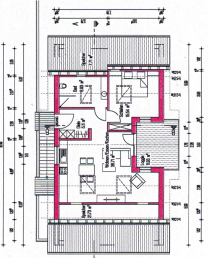
DACHGESCHOSS
