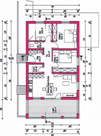
OBERGESCHOSS
