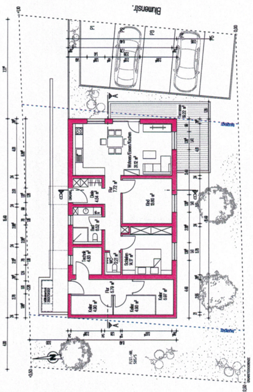
ERDGESCHOSS
