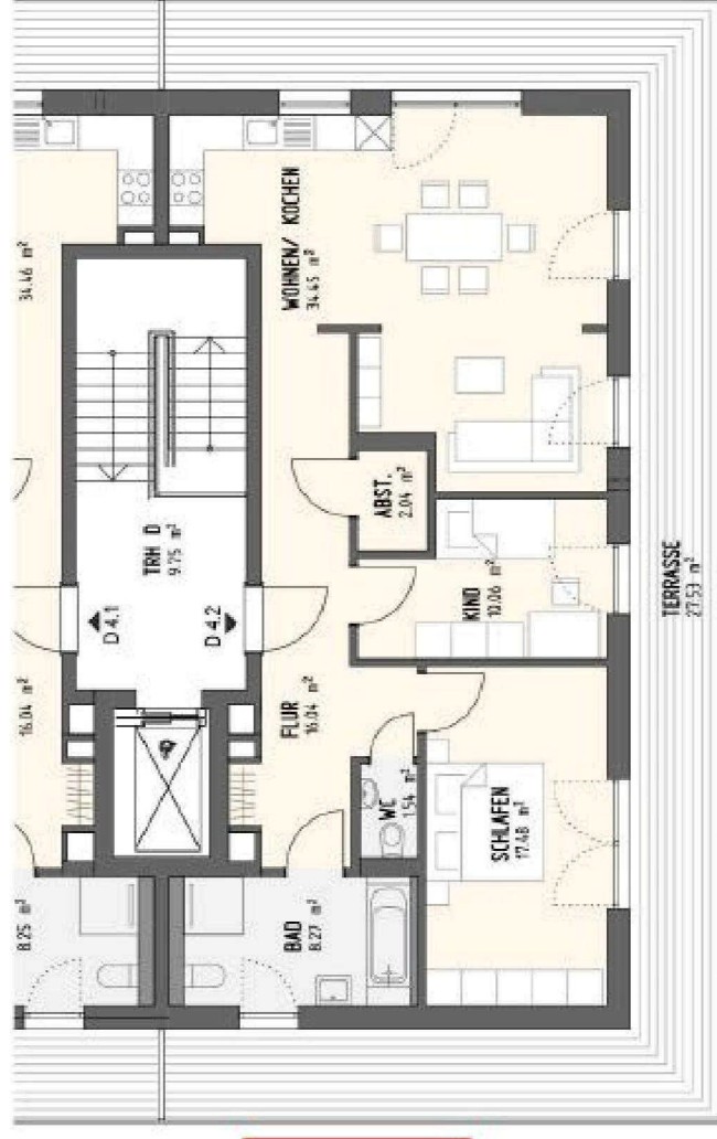
WOHNUNG D 4.2 (4 ZIMMER) M 1:100
