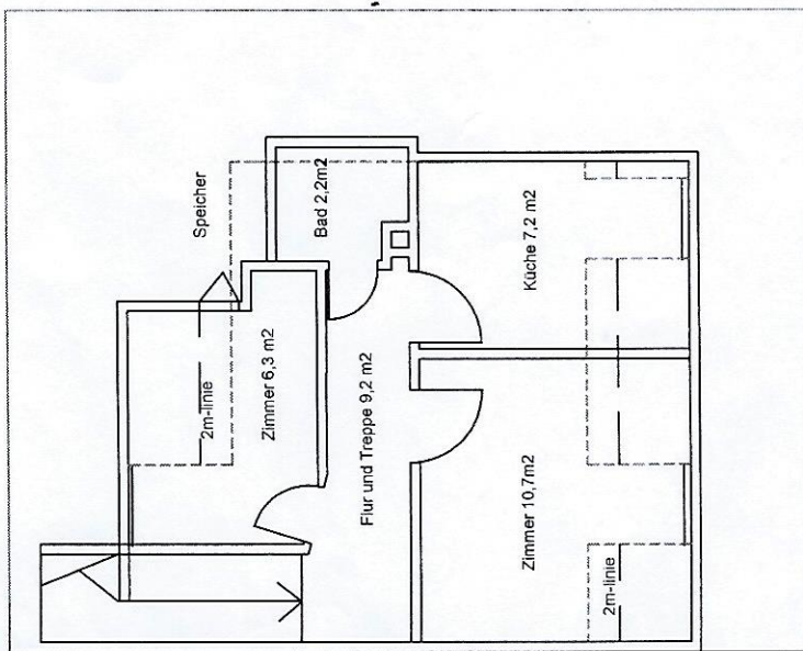
Gebäude Leibnitzstraße 14, Burghausen Grundriss DG, Wohnung ges. 36,5 m 2 , M 1:100
