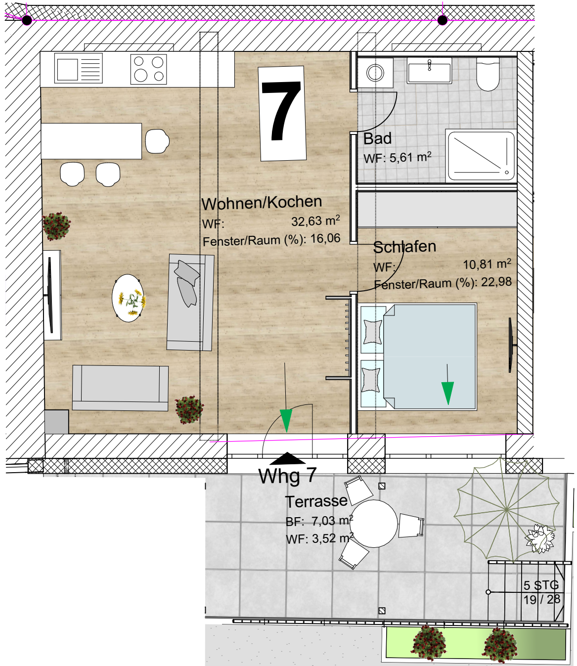
Wohnbeispiel Wohnfl. 52,57m 2
