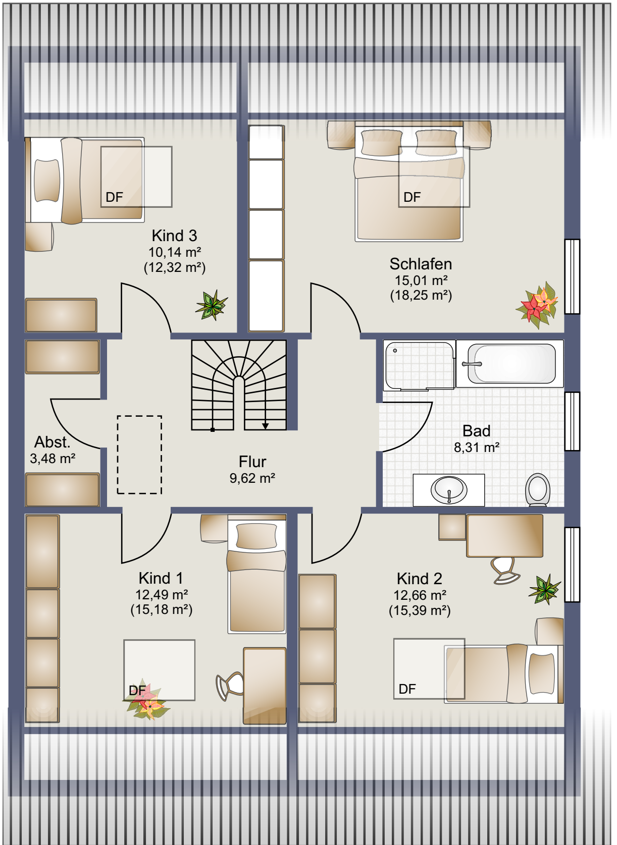
Dachgeschoss
