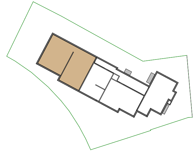
GRUNDRISS OBERGESCHOSS 2 ÜBERSICHT
