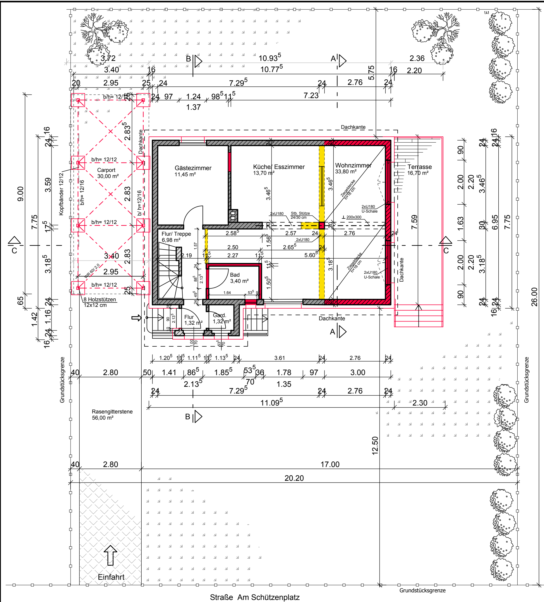
Grundriss Erdgeschoss M 1:100
