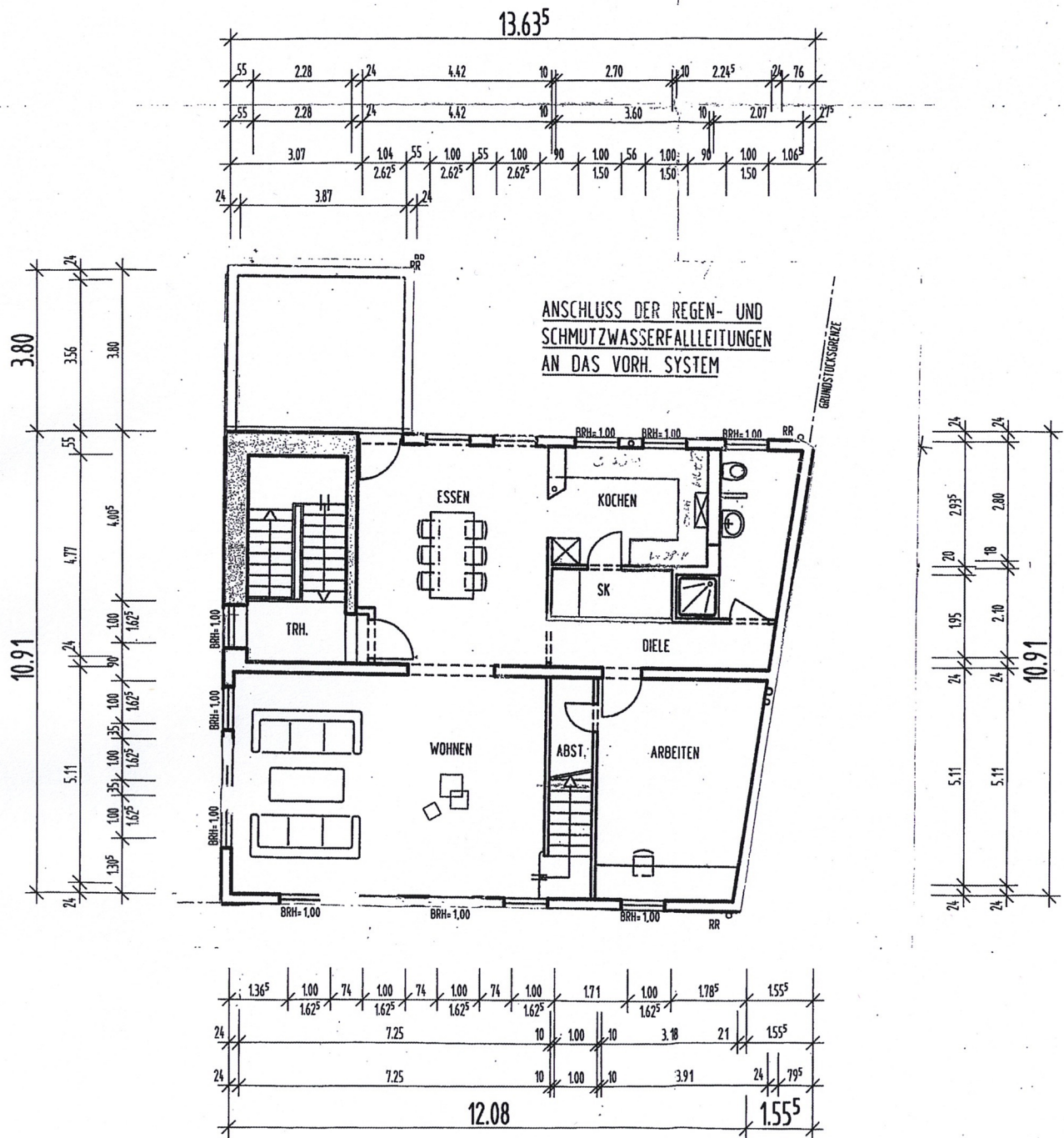
GRUNDRISS OBERGESCHOSS M 1:100
