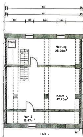
Kellergeschoss
