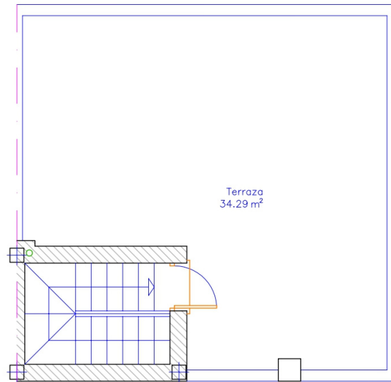
PLANTA 1, S.C.=42.41
