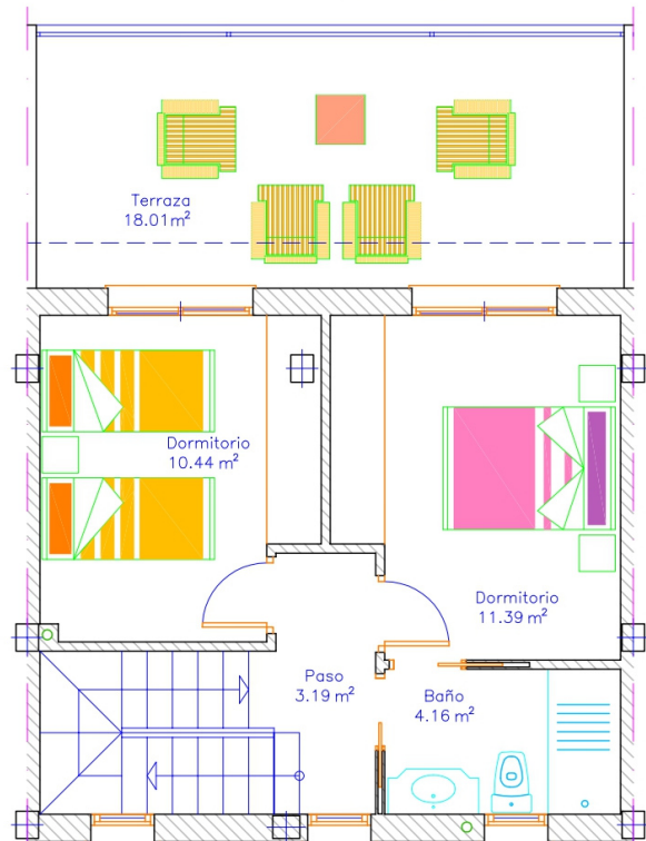
PLANTA 1, S.C.=42.41
