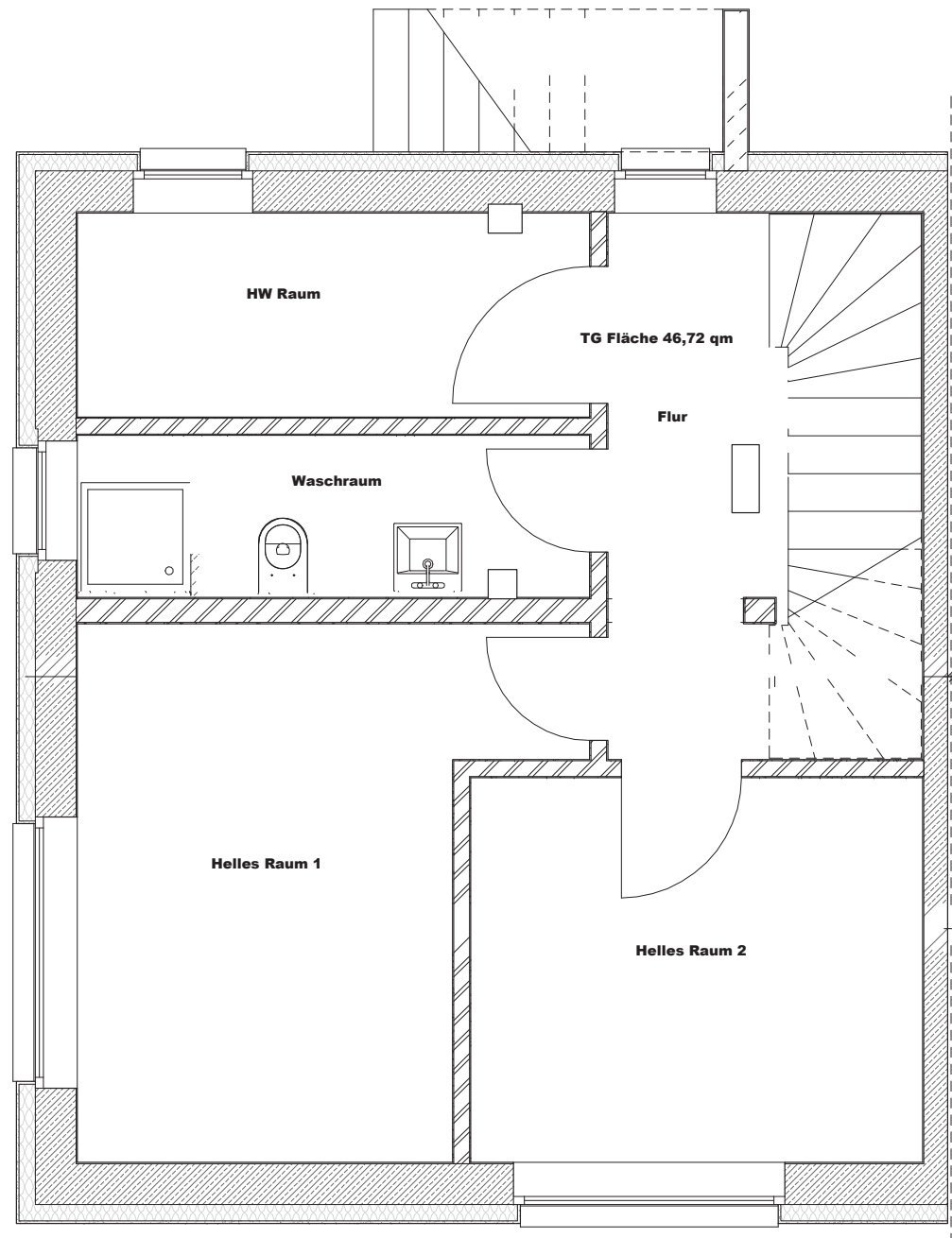
KELLER LAYOUT
