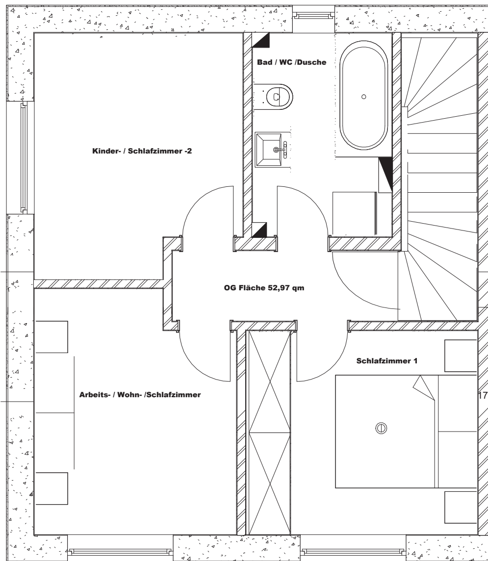
OBERGESCHOß LAYOUT
