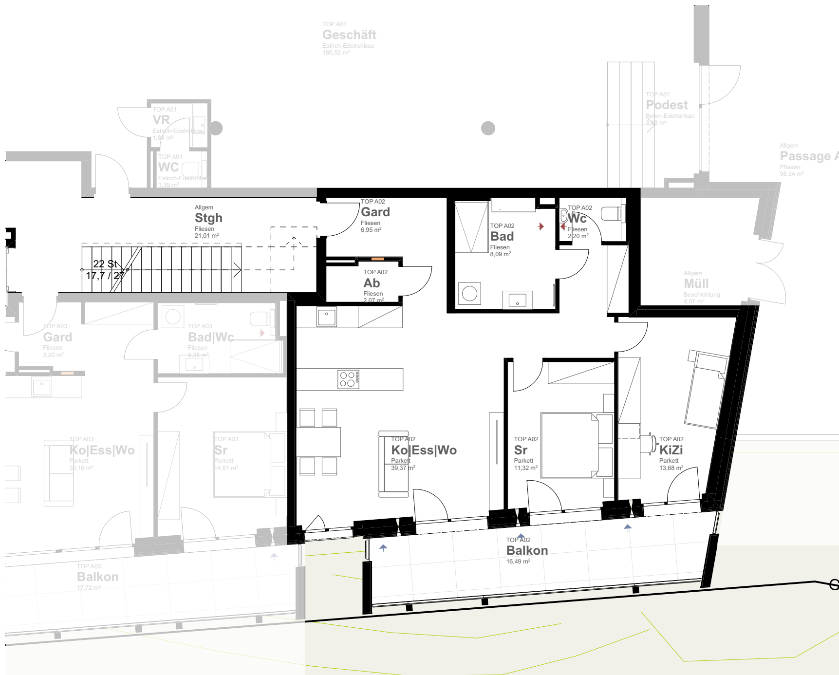
TopA02 - Haus A - EG
