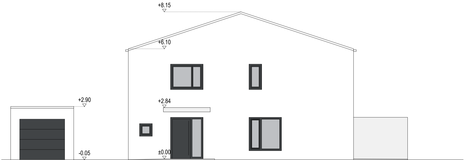
Ansicht West
